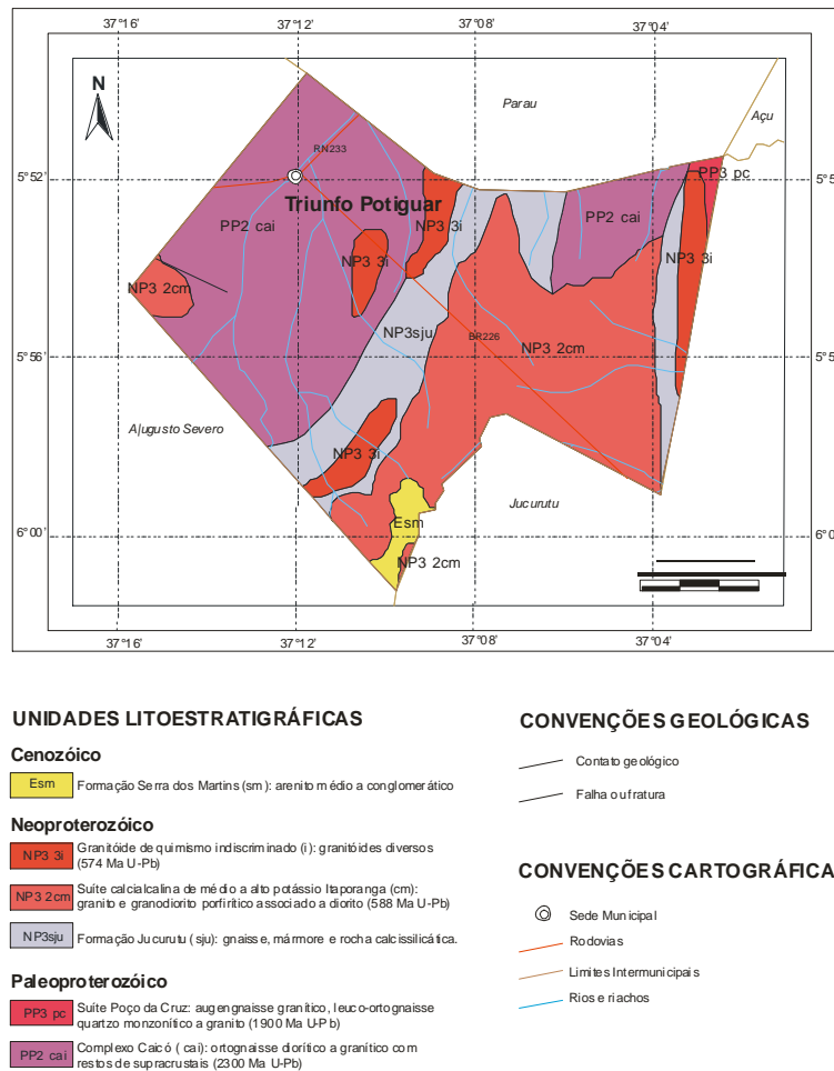
Figura 3 - Mapa Geológico
