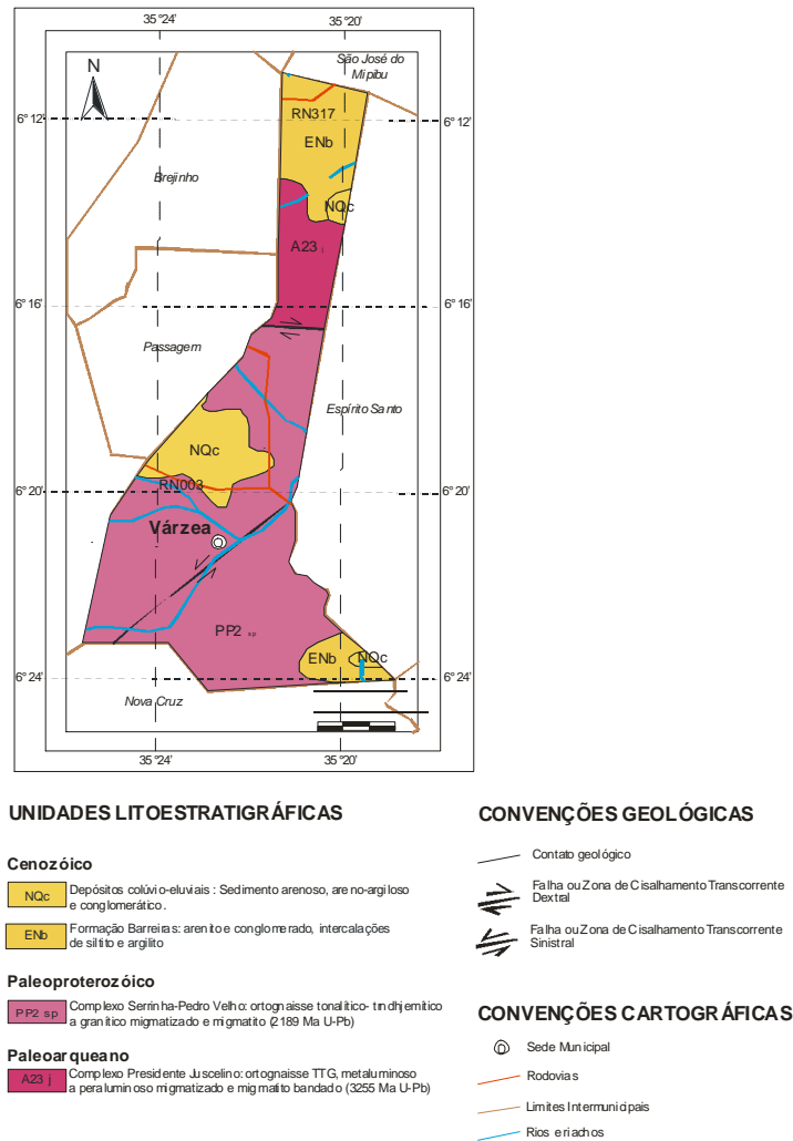
Figura 3 - Mapa Geológico
