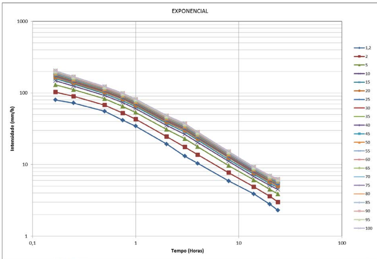
Figura 02 – Curvas intensidade-duração-frequência
