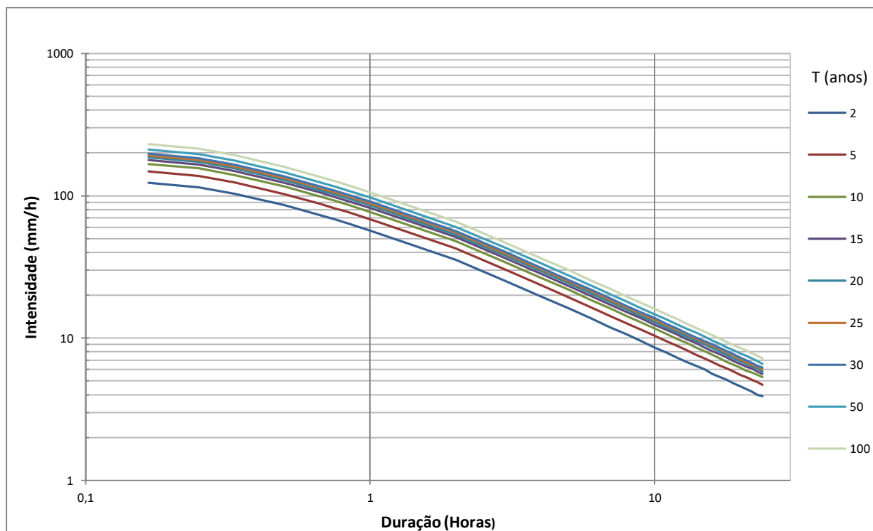
Figura 02 – Curvas intensidade-duração-frequência
