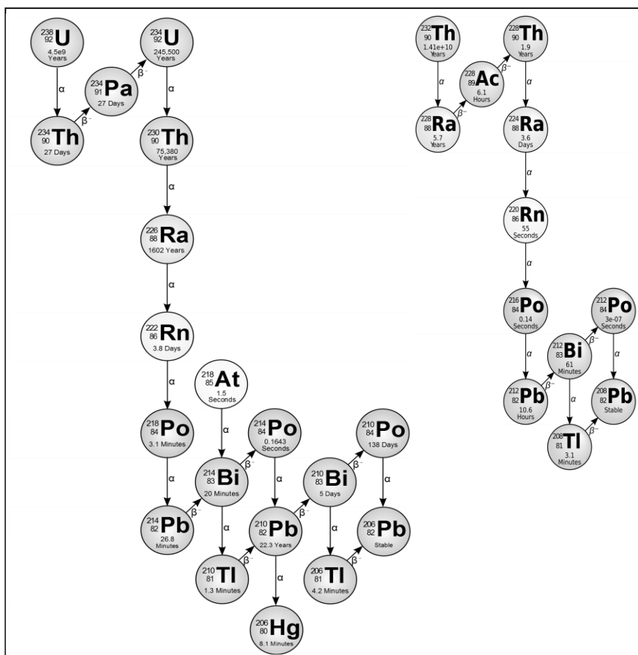
Figura 4: Séries de decaimento \alpha e \beta dos elementos ^{238}\text{U} e ^{232}\text{Th} até atingir a estabilidade. (Fonte: https://netnature.wordpress.com/2014/05/22/metodo-de-datacao-a-geologia-enterrando-a-terra-jovem/ , último acesso 11/12/2019).
