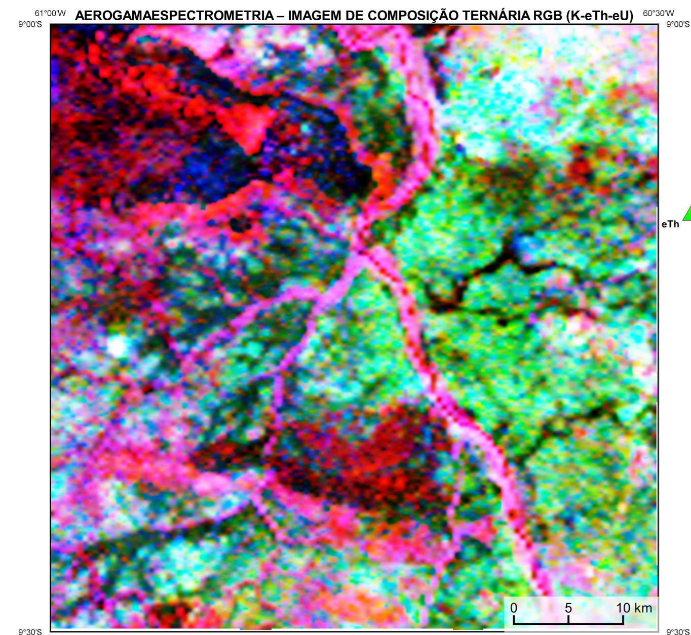
Mostra a variação das concentrações relativas dos três radioelementos relacionando-os com as cores vermelho (K-red), verde (G-green) (Th) e azul (B-blue) (eU). O espectro de cores varia do branco, quando coincidente as máximas concentrações relativas nos três radioelementos, até o preto, para os mínimos valores relativos.
