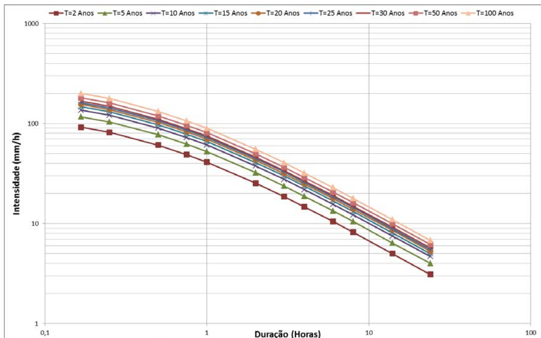
Figura 02 – Curvas intensidade-duração-freqüência
