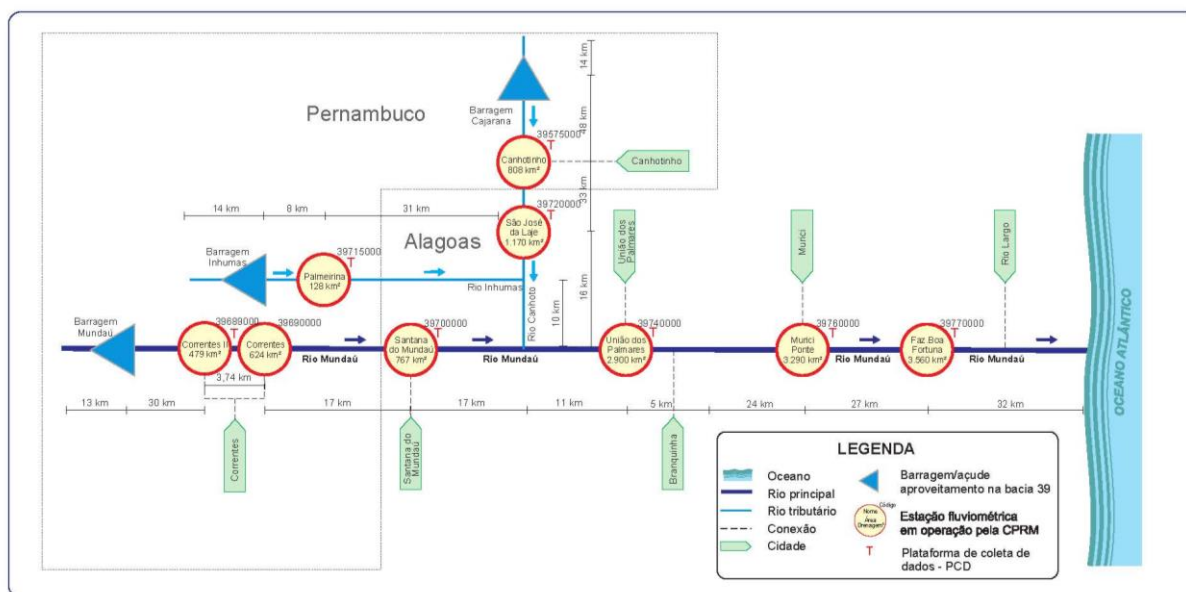
Figura 2 - Diagrama unifilar da bacia do rio Mundaú.
