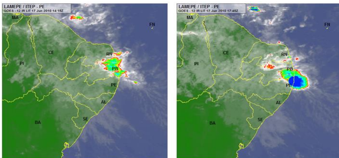
Figura 6 - Distúrbio da onda de leste, adentrando o continente no dia 17 de junho de 2010, às 11:15h e 14:45h (SANTOS, 2013).
