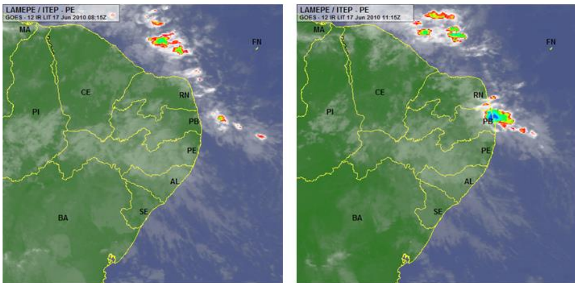
Figura 5 - Distúrbio da onda de leste, adentrando o continente no dia 17 de junho de 2010, às 05:15h e 08:15h (SANTOS, 2013).
