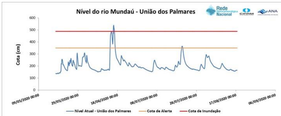
Figura 20 – Gráfico do nível do rio Mundaú em União dos Palmares – AL no período de operação de 2020.
