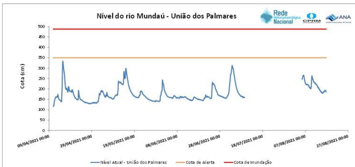
Figura 19 - Nível do rio Mundaú no município de União dos Palmares – AL no período de 10/04/21 à 16/08/21.
