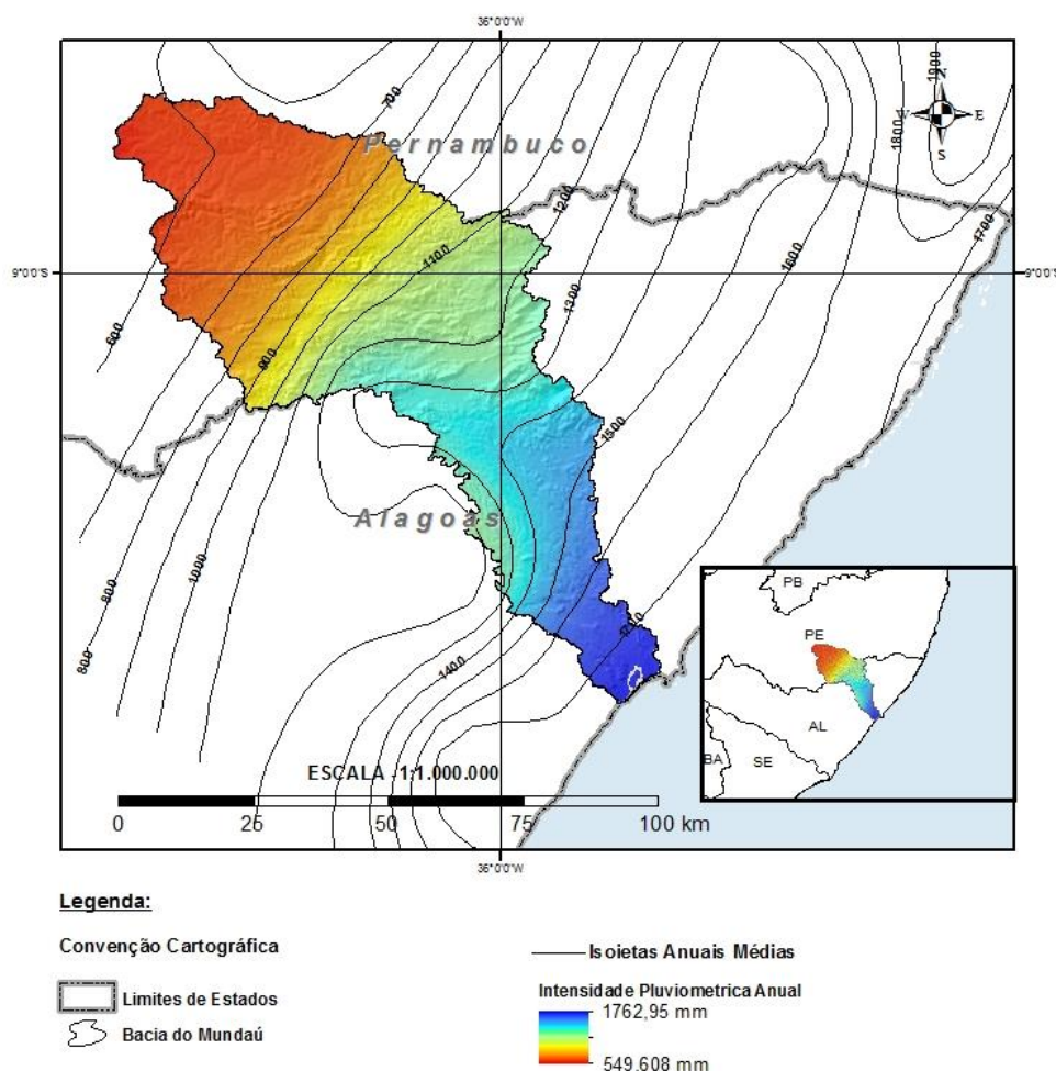
Figura 3 - Isoietas Anuais Médias, período de 1977 – 2006.
