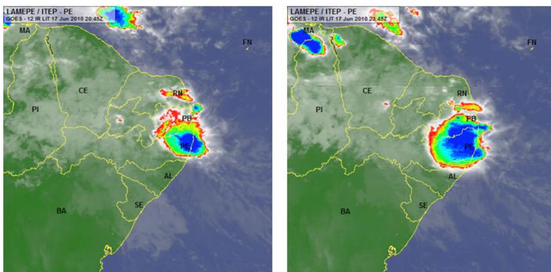
Figura 7 - Distúrbio da onda de leste, adentrando o continente no dia 17 de junho de 2010, às 17:45h e 20:45h (SANTOS, 2013).
