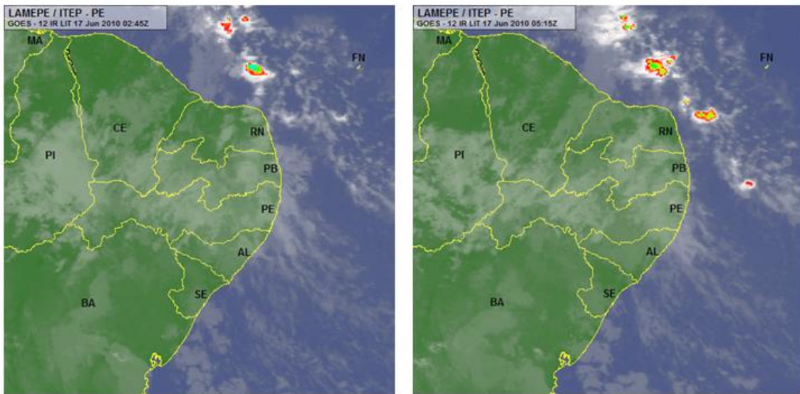
Figura 4 - Distúrbio da onda de leste, adentrando o continente nos dias 16 e 17 de junho de 2010, às 23:45h e 02:15h, respectivamente (SANTOS, 2013).
