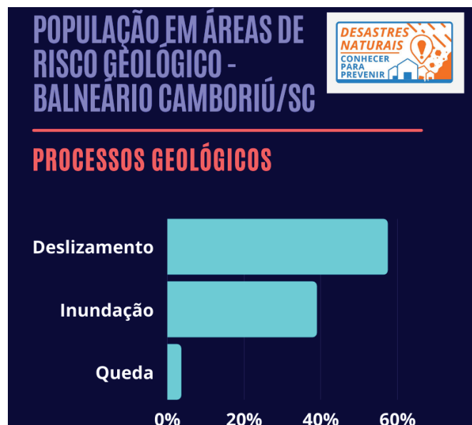
Figura 07 - Processos geológicos associados às áreas de risco
