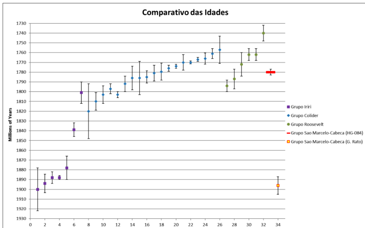
Figura 47: Gráfico comparativo da idade do Grupo São Marcelo-Cabeça obtida neste estudo (#33) com as existentes na literatura para o próprio São Marcelo-Cabeça (#34), o Grupo Iriri (#s 1 a 7), o Grupo Colíder (#s 8 a 26), e para o Grupo Roosevelt (#s 27 a 32). Referências na tabela 11.
