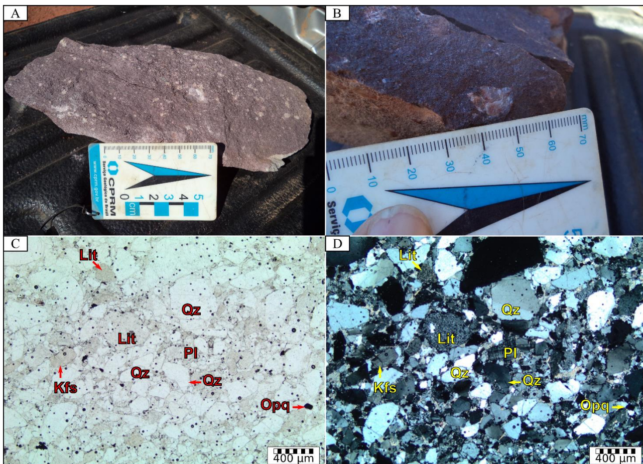
Figura 25: (A) Aspecto macroscópico da amostra DF-247-B (meta-arenito vulcanoclástico) mostrando matriz amarronzada com litoclastos de até 1,5 cm; (B) detalhe da amostra com clasto de chert ; lâmina DF-247-B em nicóis paralelos (C) e cruzados (D), mostrando os estratos mal selecionados, granocrescentes de baixo para cima da foto.
