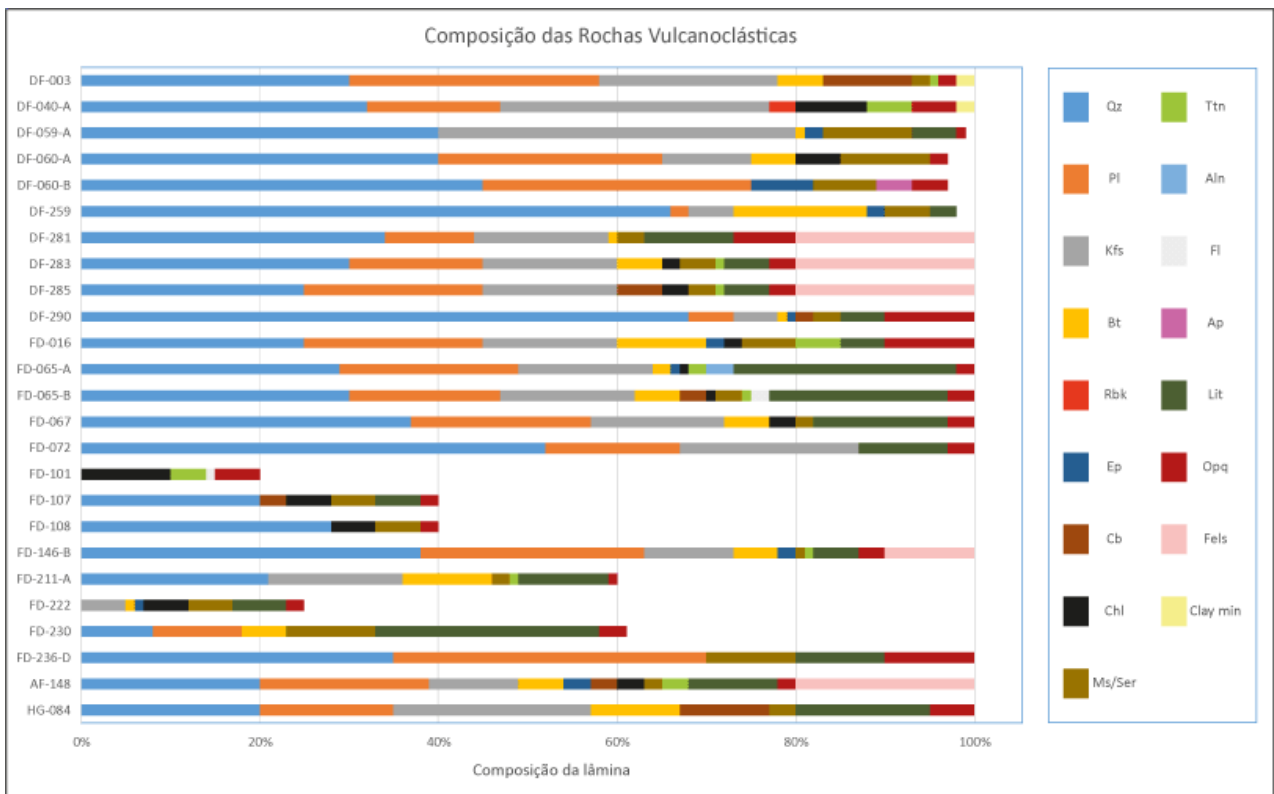
Figura 29: Quadro comparativo das composições das amostras do grupo 2. As amostras DF-003 a FD-236-D são rochas do Grupo Roosevelt, e as amostras AF-148 a HG-084 são rochas do Grupo São Marcelo-Cabeça. Valores na tabela 4.
