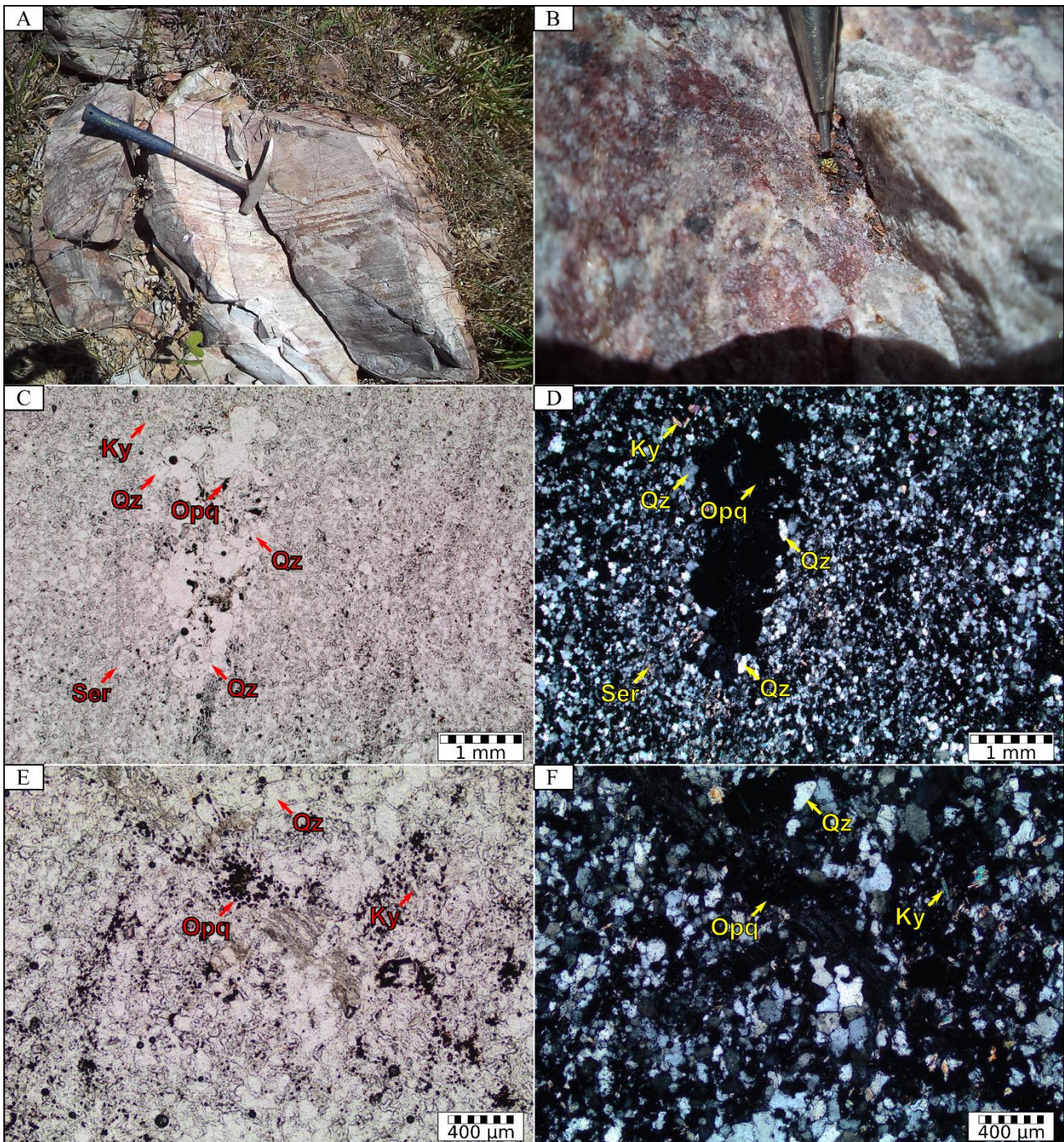
Figura 8: (A) Afloramento da amostra DF-185-A (cianita-quartzito); (B) calcopirita rodeada por hidróxido de ferro, (C e D) microfotografias da lâmina mostrando textura granoblástica fina e os mosaicos de quartzo poligonal; (E e F) detalhes dos aglomerados de minerais opacos e dos cristais de quartzo.
