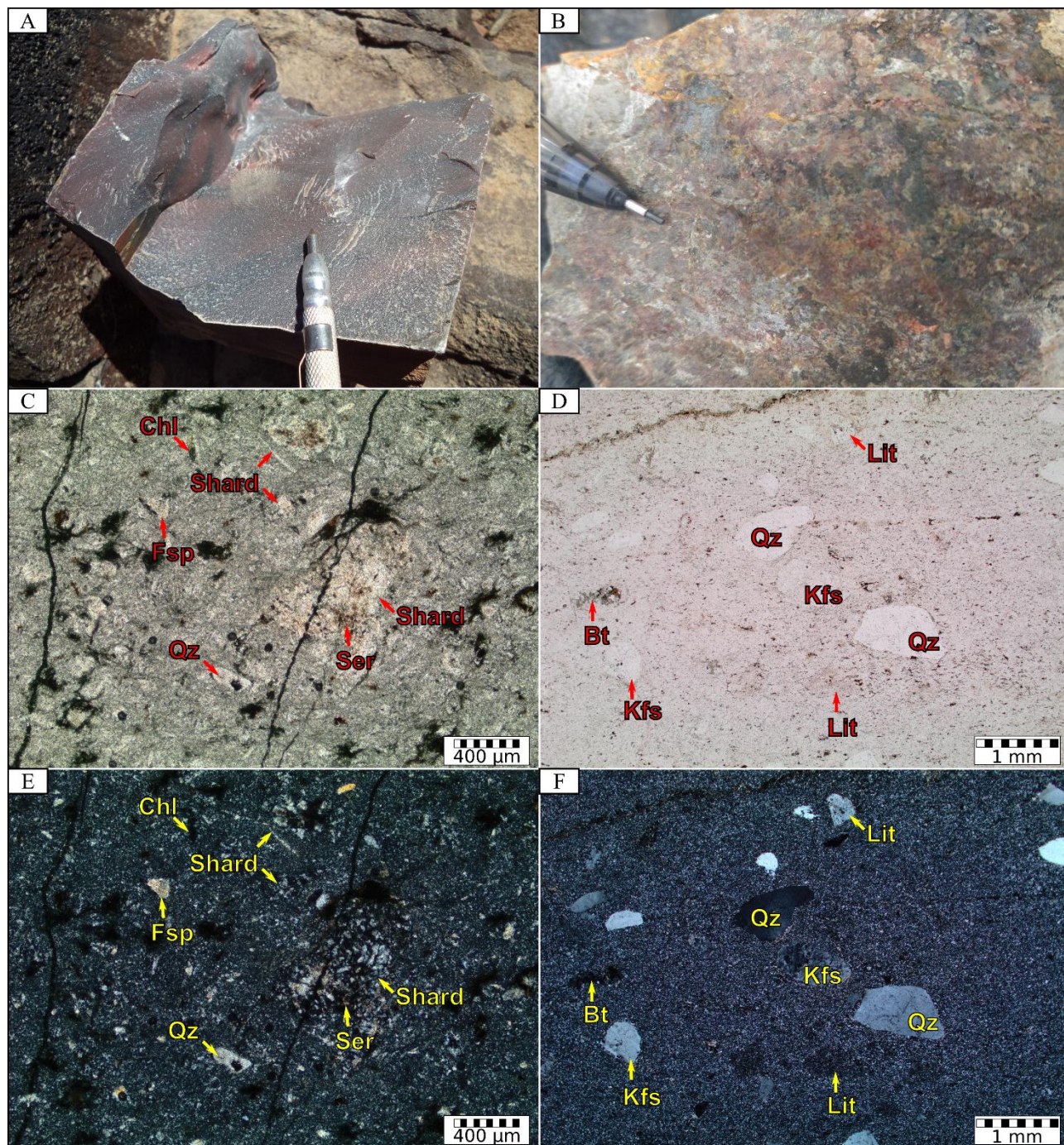
Figura 22: Aspectos macroscópicos e microscópicos das amostras de metatufo cinerítico FD-107 (A, C e E) e FD-222 (B, D e F); (A) Amostra FD-107 silicificada, mostrando estrutura maciça; (B) amostra FD-222 mostrando alteração hidrotermal sofrida da rocha; lâmina FD-107 em nicóis paralelos (C) e cruzados (E), mostrando vários formatos de shards devitrificados e metassomatizados; lâmina FD-222 em nicóis paralelos (D) e cruzados (F), mostrando matriz microgranular com textura microporfírica.
