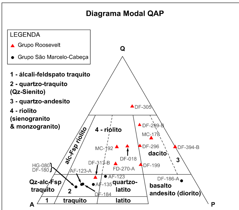
Figura 30: Gráfico QAP com as estimativas composicionais do grupo 1. Em parênteses estão os nomes das rochas plutônicas equivalentes das vulcânicas.
