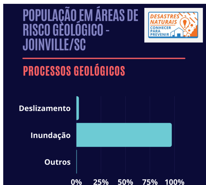
Figura 07 - Processos geológicos associados às áreas de risco
