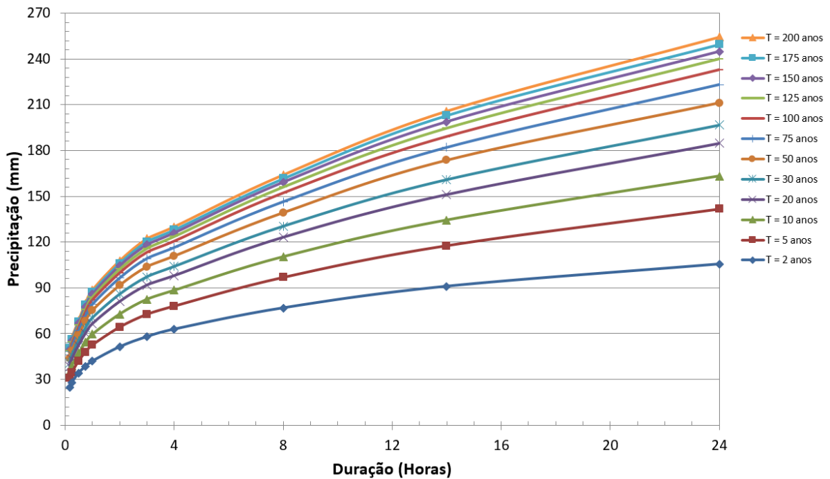
Figura 04 – Curvas Altura-Duração-Freqüência (PA de 1700mm).
