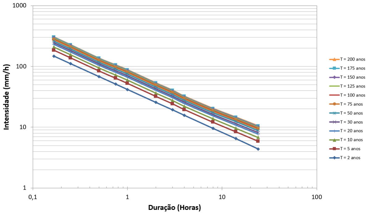
Figura 03 – Curvas Intensidade-Duração-Freqüência (PA de 1700mm).
