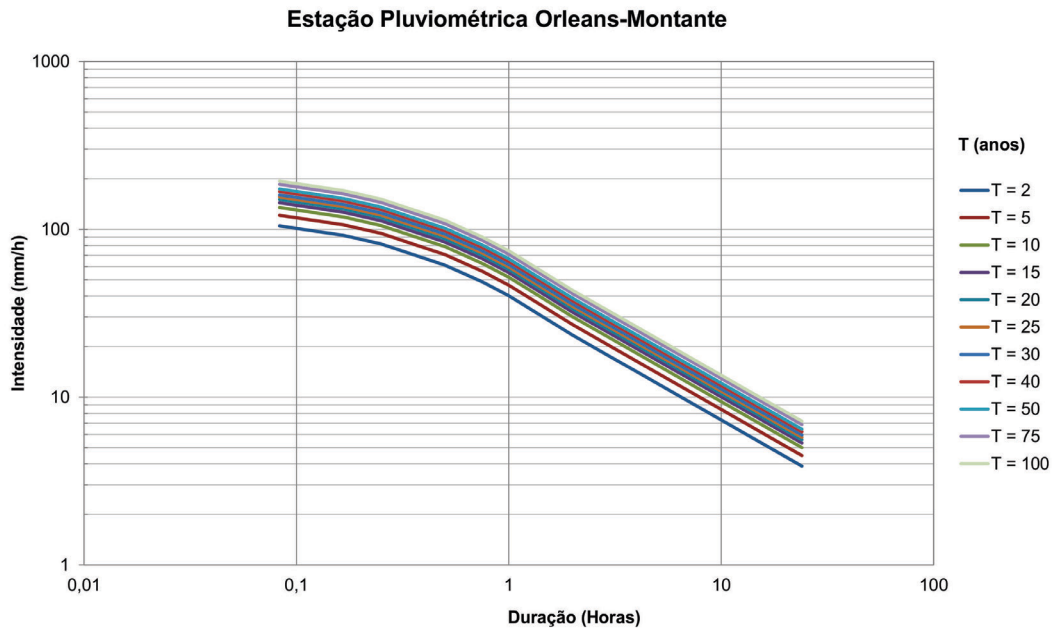
Figura 02 - Curvas intensidade-duração-frequência
