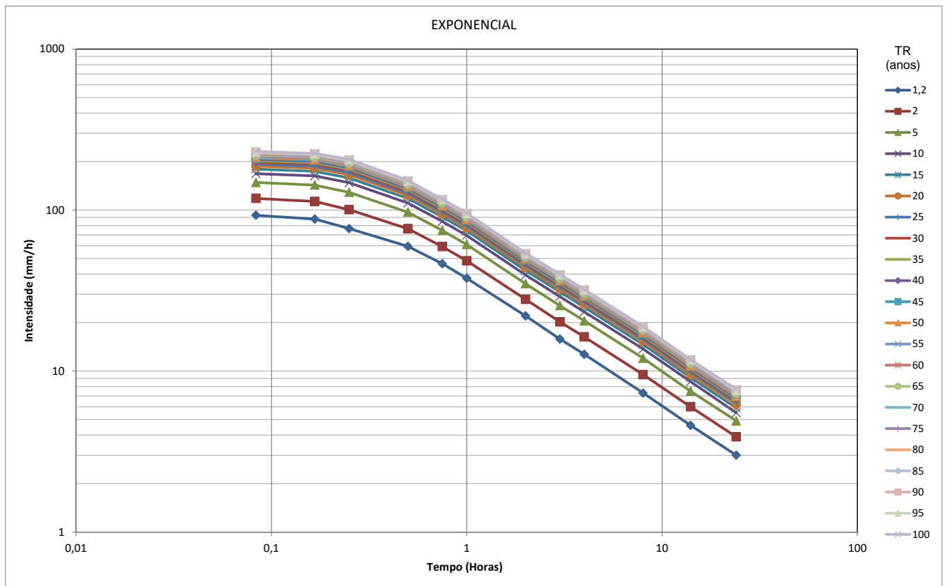
Figura 02 – Curvas intensidade-duração-frequência
