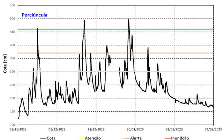
Figura 10 - Cotagrama de Porciúncula entre 01/11/2022 e 31/03/2023: cota (linha preta), cota de atenção (linha amarela), cota de alerta (linha laranja) e cota de inundação (linha vermelha).
