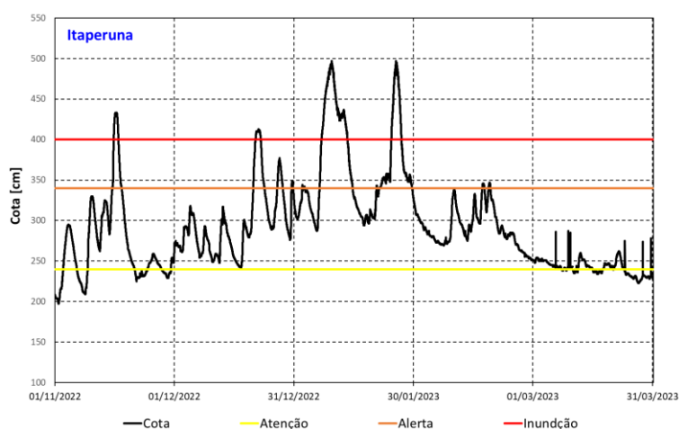
Figura 11 - Cotagrama de Itaperuna entre 01/11/2022 e 31/03/2023: cota (linha preta), cota de atenção (linha amarela), cota de alerta (linha laranja) e cota de inundação (linha vermelha).
