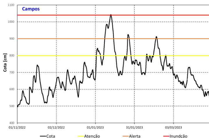
Figura 13 - Cotagrama de Campos entre 01/11/2022 e 31/03/2023: cota (linha preta), cota de atenção (linha amarela), cota de alerta (linha laranja) e cota de inundação (linha vermelha).
