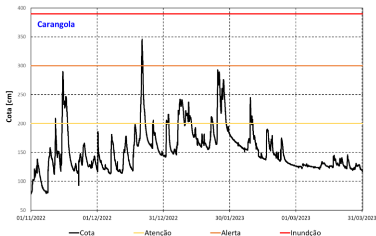
Figura 9 – Cotagrama de Carangola entre 01/11/2022 e 31/03/2023: cota (linha preta), cota de atenç o (linha amarela), cota de alerta (linha laranja) e cota de inundaç o (linha vermelha).
