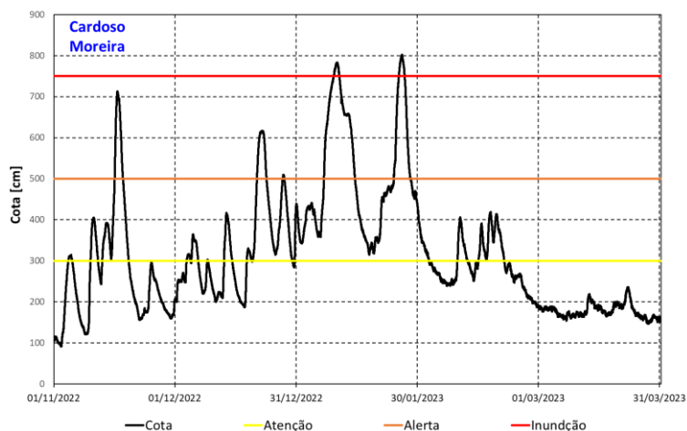
Figura 12 - Cotagrama de Cardoso Moreira entre 01/11/2022 e 31/03/2023: cota (linha preta), cota de atenção (linha amarela), cota de alerta (linha laranja) e cota de inundação (linha vermelha).
