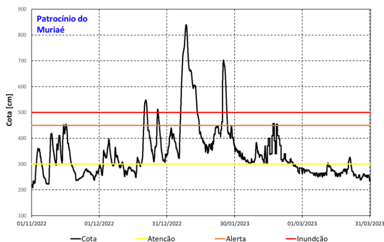
Figura 8 – Cotagrama de Patroc nio do Muria  entre 01/11/2022 e 31/03/2023: cota (linha preta), cota de atenç o (linha amarela), cota de alerta (linha laranja) e cota de inundaç o (linha vermelha).
