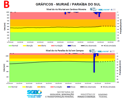
Figura 3 - Páginas do modelo do boletim extraordinário do SAH-Muriaé. (A) Tabela com dados hidrológicos das estações. (B) Gráficos com cotogramas, pluviogramas e cotas simuladas para estações do SAH-Muriaé.
