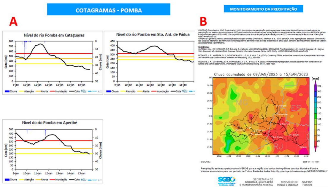
Figura 4 - Páginas do Boletim de Monitoramento. (A) Gráficos com o comportamento da cota e da precipitação das estações do SAH-Pomba. (B) Imagem de precipitação estimada pelo produto MERGE.
