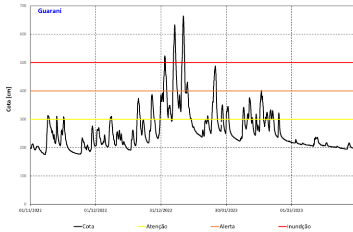
Figura 8 – Cotagrama de Guarani entre 01/11/2022 e 31/03/2023: cota (linha preta), cota de atenção (linha amarela), cota de alerta (linha laranja) e cota de inundação (linha vermelha).
