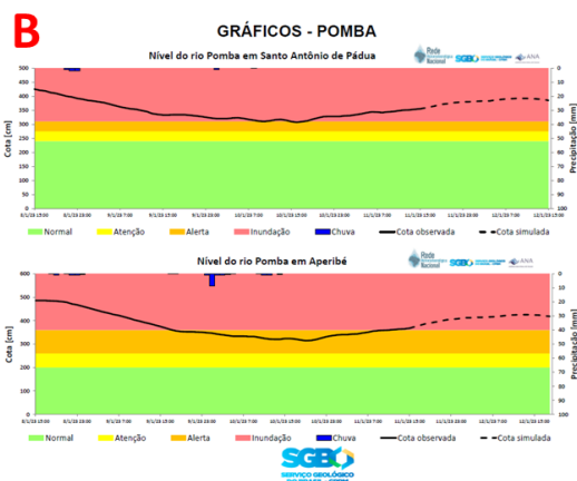
Figura 3 - Páginas do modelo do boletim de alerta do SAH-Pomba. (A) Tabela com dados hidrológicos das estações. (B) Gráficos com cotogramas, pluviogramas e cotas simuladas para estações do SAH-Pomba.
