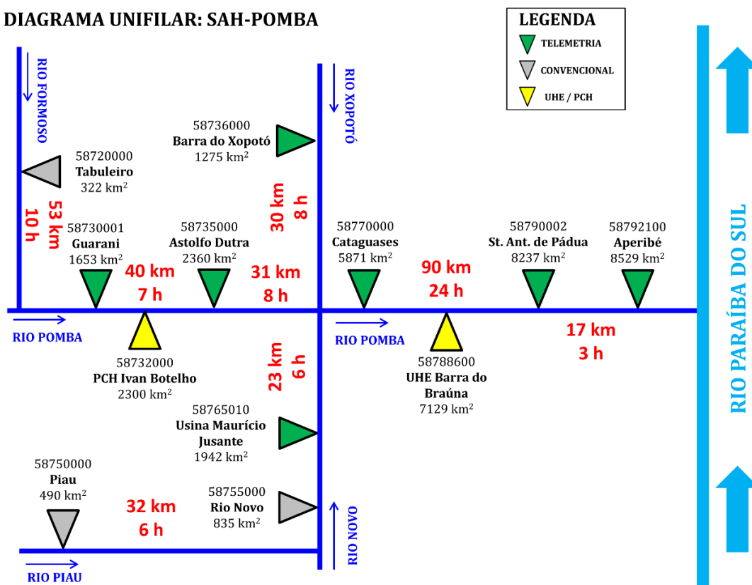
Figura 2 – Diagrama unifilar do SAH-Pomba.
