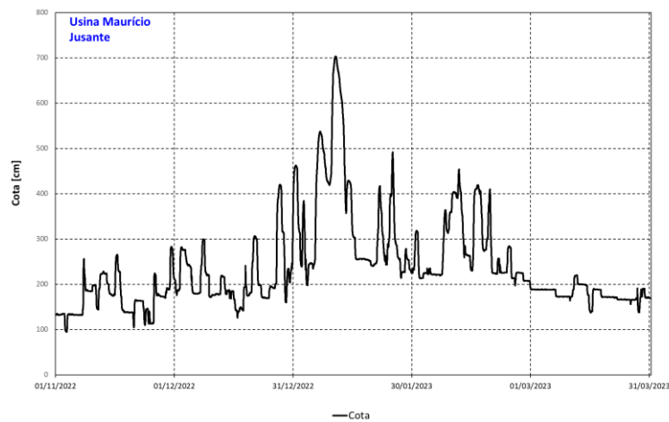
Figura 9 – Cotagrama de Usina Maurício Jusante entre 01/11/2022 e 31/03/2023: cota (linha preta), cota de atenção (linha amarela), cota de alerta (linha laranja) e cota de inundação (linha vermelha).
