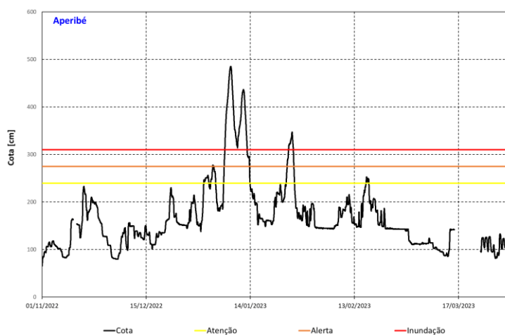
Figura 13 - Cotagrama de Aperibé entre 01/11/2022 e 31/03/2023: cota (linha preta), cota de atenção (linha amarela), cota de alerta (linha laranja) e cota de inundação (linha vermelha).
