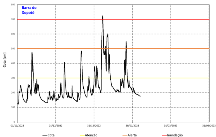
Figura 10 - Cotagrama de Barra do Xopotó entre 01/11/2022 e 31/03/2023: cota (linha preta), cota de atenção (linha amarela), cota de alerta (linha laranja) e cota de inundação (linha vermelha).
