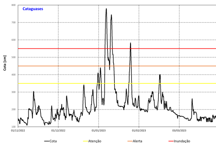
Figura 11 - Cotagrama de Cataguases entre 01/11/2022 e 31/03/2023: cota (linha preta), cota de atenção (linha amarela), cota de alerta (linha laranja) e cota de inundação (linha vermelha).
