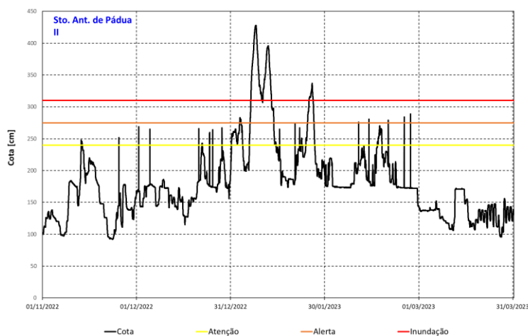
Figura 12 - Cotagrama de Santo Antônio de Pádua II entre 01/11/2022 e 31/03/2023: cota (linha preta), cota de atenção (linha amarela), cota de alerta (linha laranja) e cota de inundação (linha vermelha).
