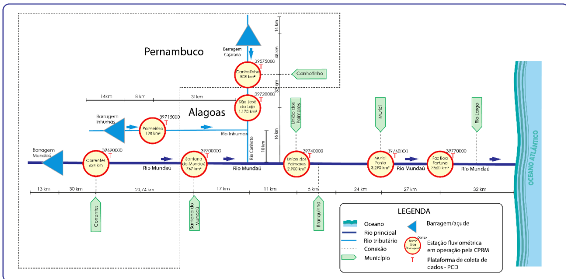
Figura 2 - Diagrama unifilar da bacía do rio Mundaú. Fonte: Elaborada pela autora.
