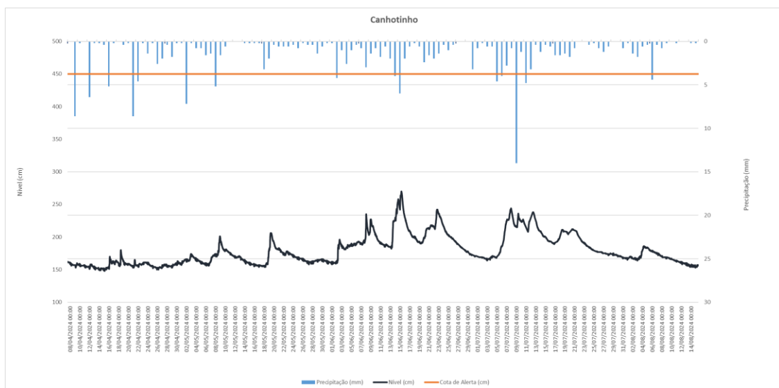
Figura 18 – Nível do rio Canhoto e precipitação na PCD da estação Canhotinho no município de Canhotinho – PE no período de 08/04/24 à 16/08/24. Fonte: Elaborada pelos autores.
