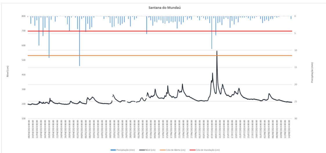
Figura 21 – Nível do rio Mundaú e precipitação na PCD da estação Santana do Mundaú no município de Santana do Mundaú – AL no período de 08/04/24 à 16/08/24. Fonte: Elaborada pelos autores.
