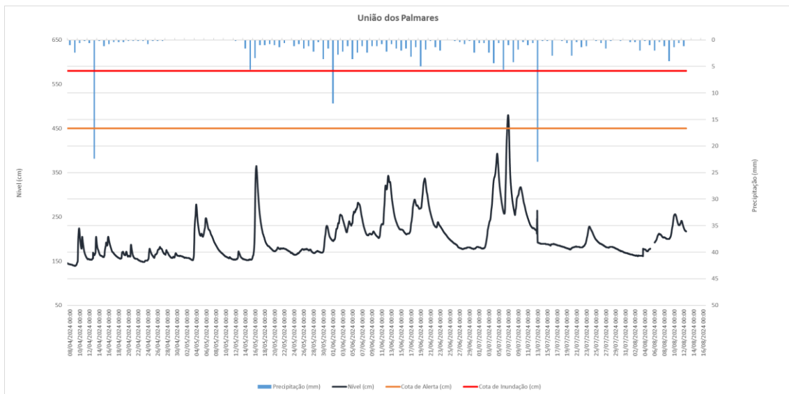
Figura 23 - Nível do rio Mundaú e precipitação na PCD da estação de União dos Palmares no município de União dos Palmares – AL no período de 08/04/24 à 16/08/24. Fonte: Elaborada pelos autores.
