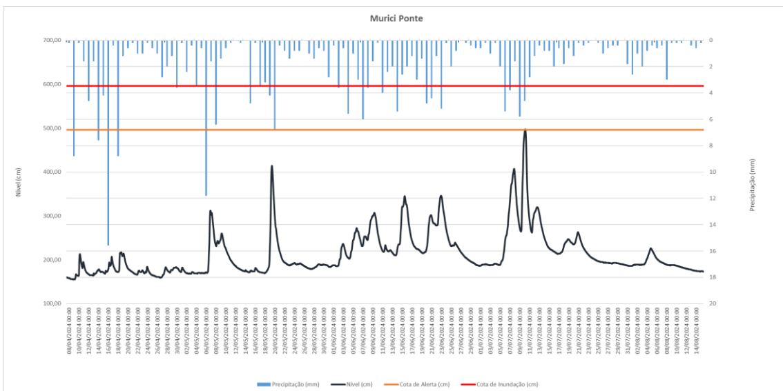
Figura 24 – Nível do rio Mundaú e precipitação na PCD da estação de Murici Ponte no município de Murici – AL no período de 08/04/24 à 16/08/24. Fonte: Elaborada pelos autores.
