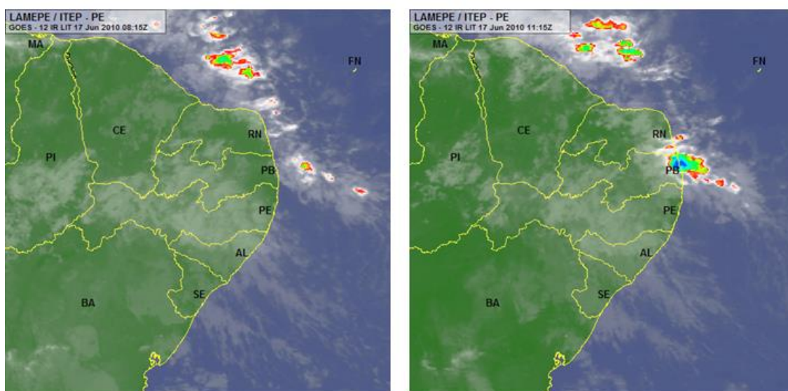
Figura 5 - Distúrbio da onda de leste, adentrando o continente no dia 17 de junho de 2010, às 05:15h e 08:15h. Fonte: Santos (2013).
