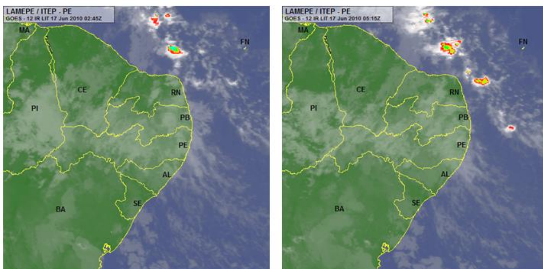
Figura 4 - Distúrbio da onda de leste, adentrando o continente nos dias 16 e 17 de junho de 2010, às 23:45h e 02:15h, respectivamente. Fonte: Santos (2013).
