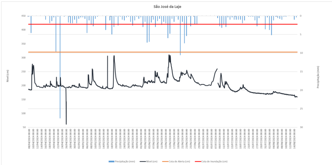
Figura 22 – Nível do rio Canhoto e precipitação na PCD da estação São José da Laje no município de São José da Laje – AL no período de 08/04/24 à 16/08/24. Fonte: Elaborada pelos autores.
