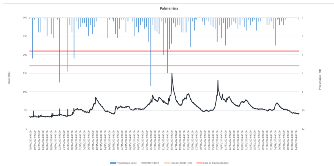
Figura 19 – Nível do rio Inhumas e precipitação na PCD da estação Palmeirina no município de Palmeirina – PE no período de 08/04/24 à 16/08/24. Fonte: Elaborada pelos autores.
