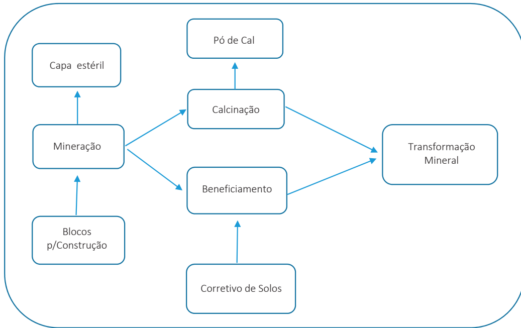
Figura 9.1 - Diagrama esquemático da cadeia produtiva de cal virgem para a construção civil. Fonte: Vargas, 2024. Adaptado.
