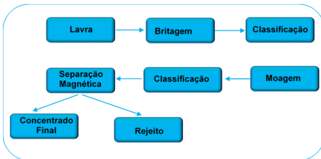
Figura 9.4 - Diagrama esquemático da cadeia produtiva do feldspato Fonte: Silva (2019). Adaptado por SGB/SEDEC (2023).
