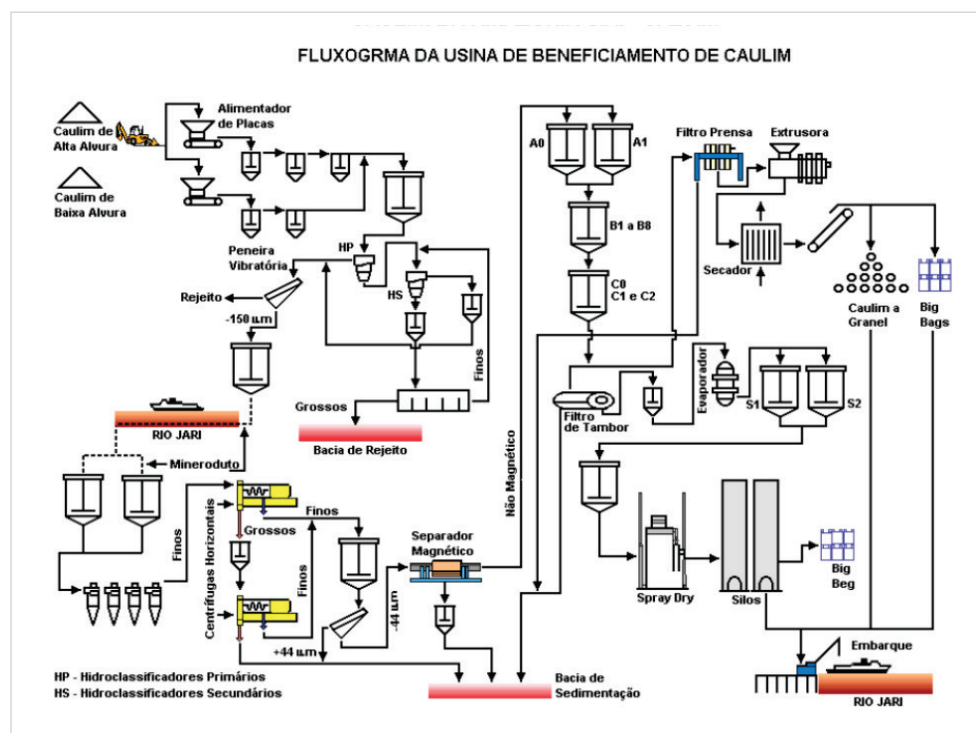
Figura 9.3 - Cadeia produtiva do caulim. Fonte: MONTE et al. (2002). Adaptado por SGB/ SEDEC (2023).
