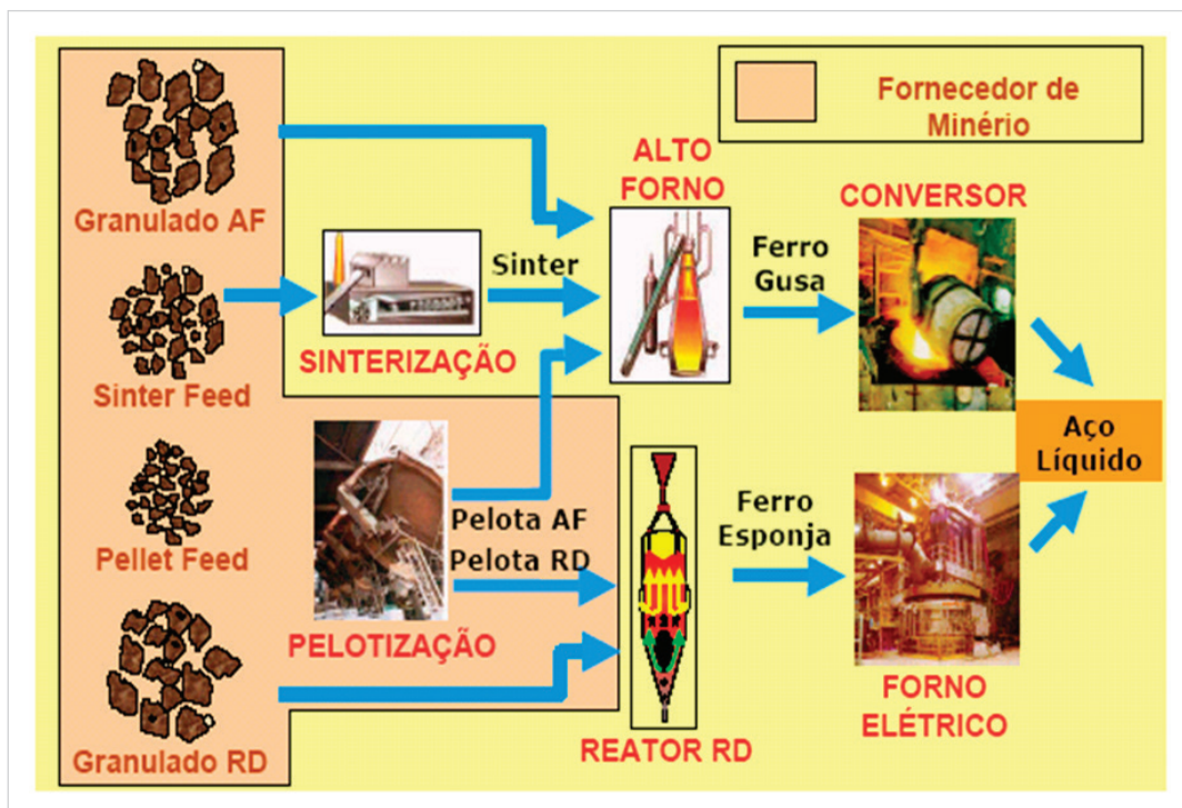
Figura 9.8 - Diagrama esquemático da cadeia do ferro. Fonte: CEFETES (2011).
