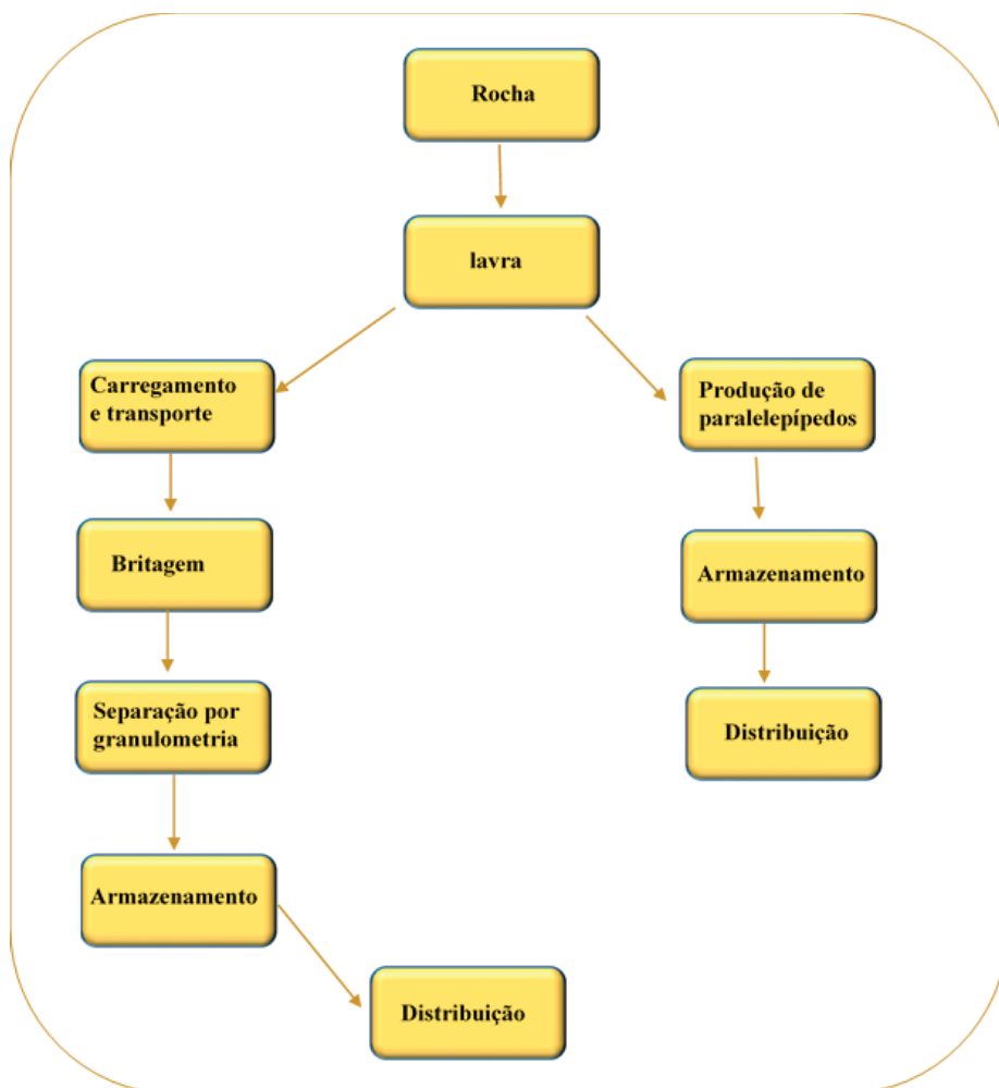
Figura 9.2 - Diagrama esquemático para a cadeia produtiva de calcário, granulados e construção civil. Fonte: Mendes (2018). Adaptado por SGB/SEDEC (2023).
