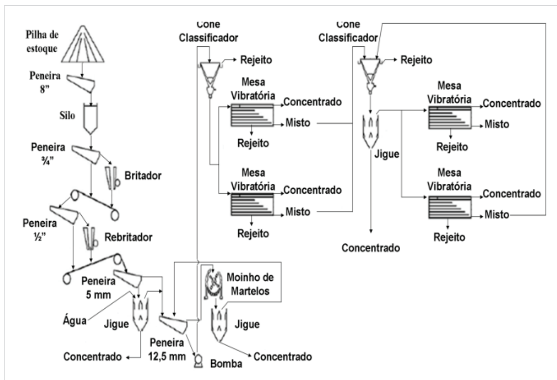
Figura 9.9 - Diagrama esquemático da cadeia produtiva da scheelita.
