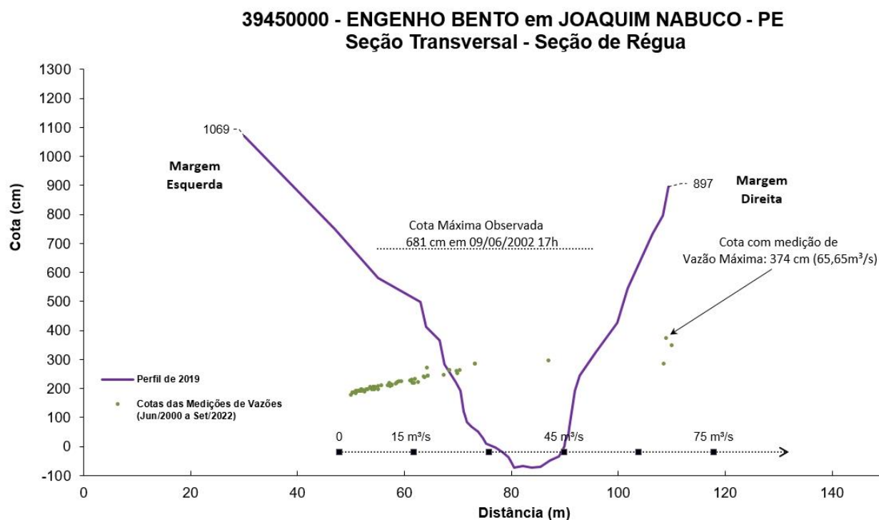
Figura 03 – Perfil da seção transversal da seção de régua de Engenho Bento. Fonte: elaborado pelos autores.
