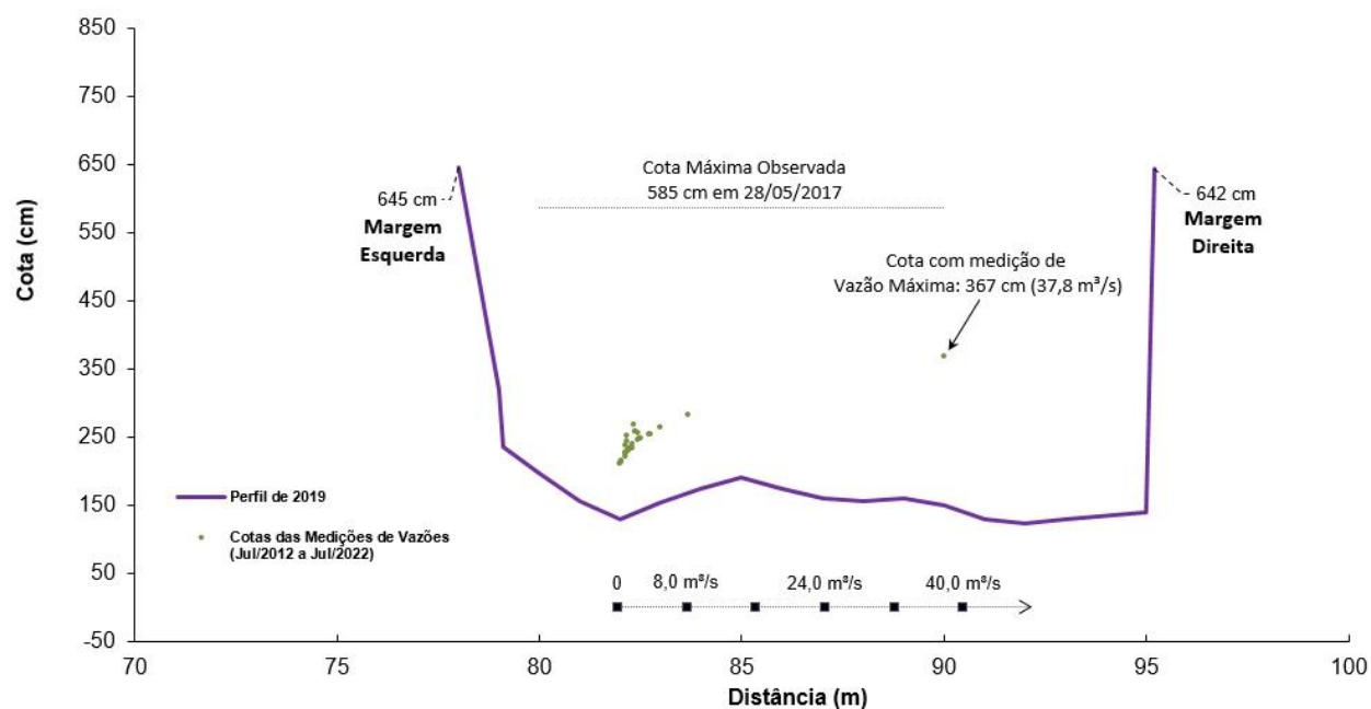
Figura 03 – Perfil da seção transversal da seção de régua de São Benedito do Sul. Fonte: elaborado pelos autores.
