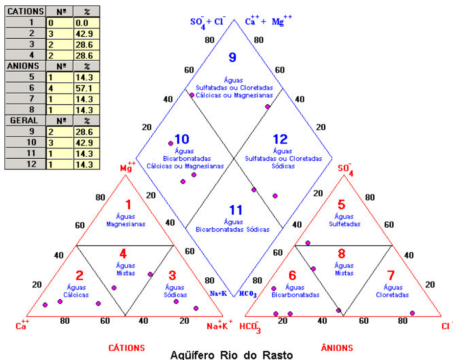
Figura 77: Diagrama de Piper para as águas do Sistema Aquífero Rio do Rasto (terço superior) e Botucatu – Aquífero Guarani.
