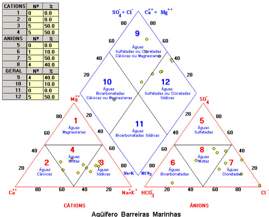
Figura 89: Diagrama de Piper para as águas do Sistema Aquífero Barreiras Marinhas com retrabalhamento eólico.
