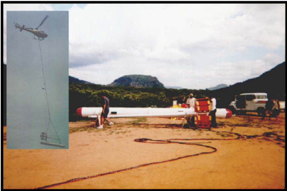
Figura 1.3 – Plataforma utilizada no aerolevante do PROASNE. Detalhe do helicóptero e do bird que contém os sensores eletromagnético e magnético. O sensor VLF (no detalhe da foto) situava-se preso ao cabo à meia distância entre a aeronave e o bird . (Lasa, 2001).
