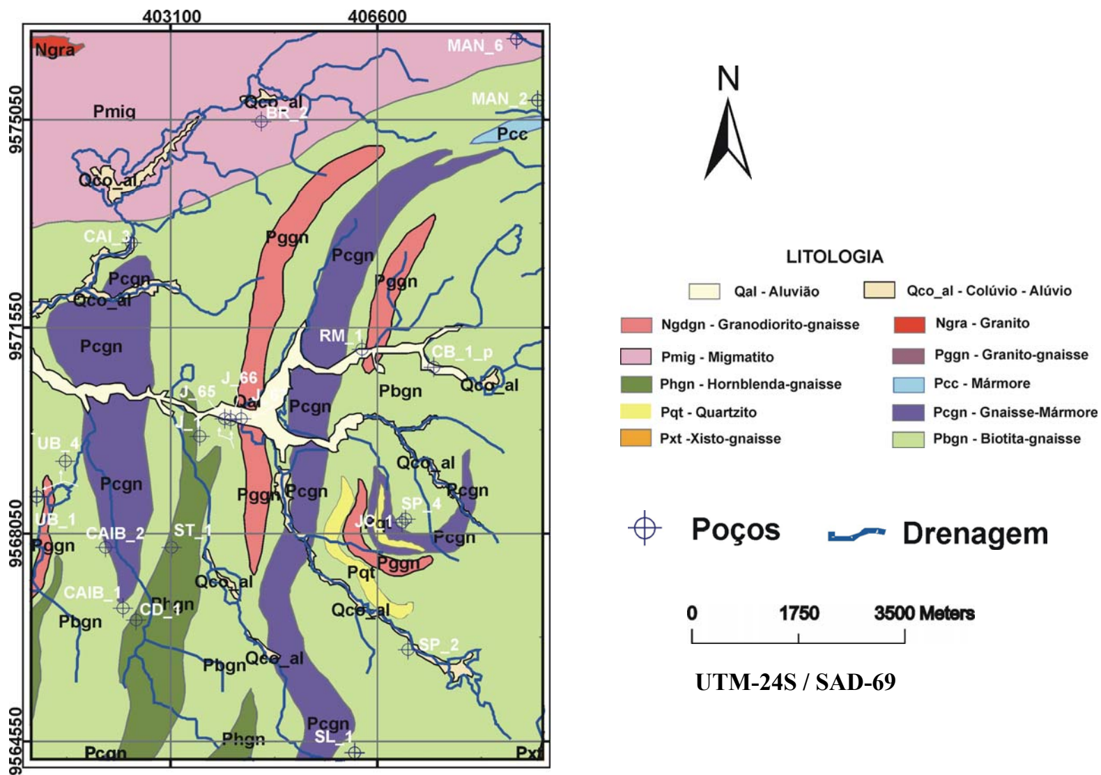
Figura 2.5 - Mapa geológico simplificado da área de estudo de Juá, Irauçuba-CE. Modificado de Souza Filho (1998).
