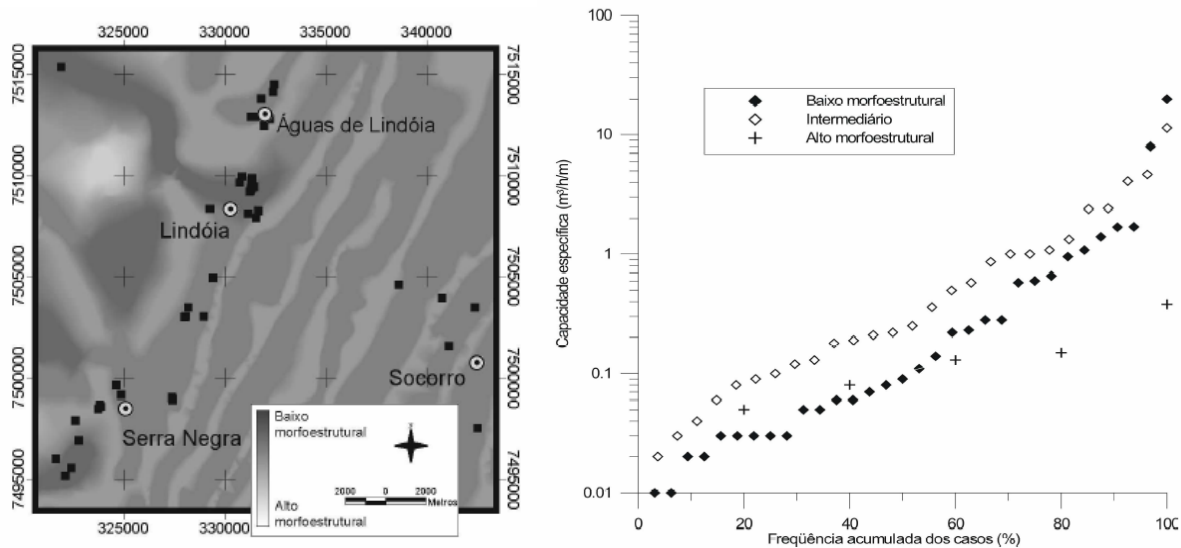
Figura 1.6 - Localização de poços e a relação positiva da produtividade com baixo morfoestrutural no cristalino de São Paulo (Mandrucci, 2003).
