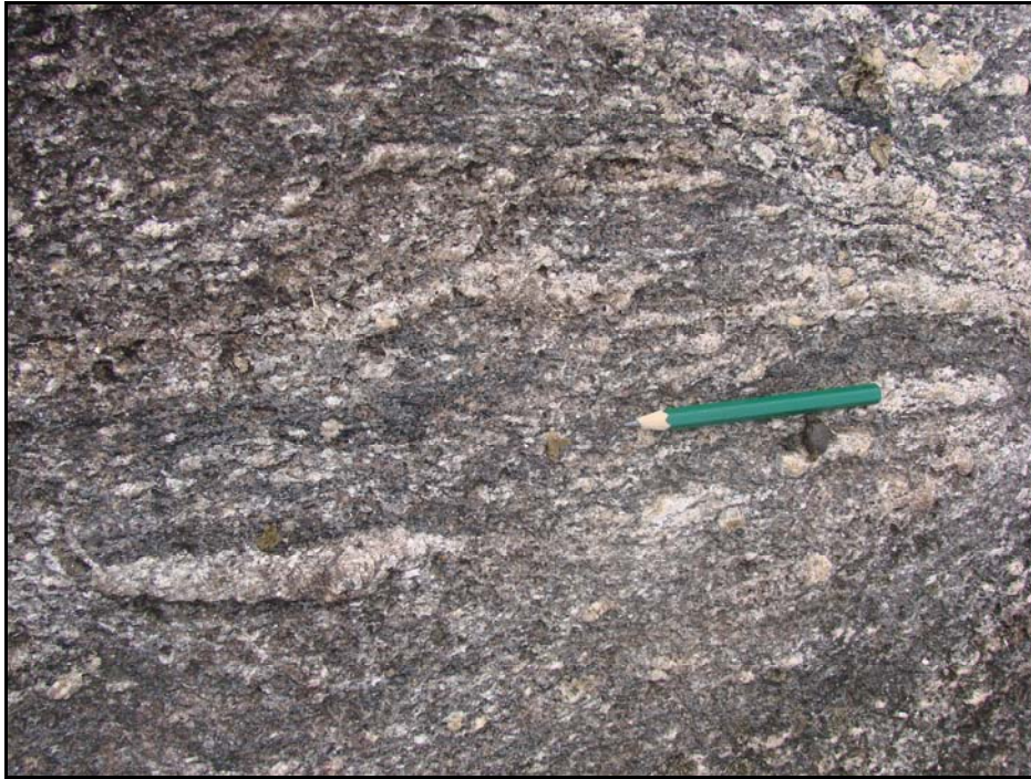
Figura 14. Textura protomilonítica do biotita-granada-Gnaiss.
