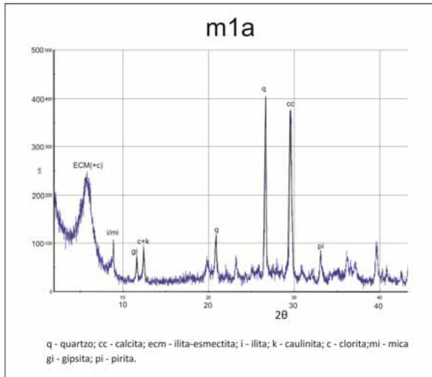
Figura 90 - Difratoograma do ritmito argilo-carbonático, microfácies m1a, da UC1 (85,56-85,64m), do poço estratigráfico 2-JSN-01-PE (Vortisch et al. , 2011).
