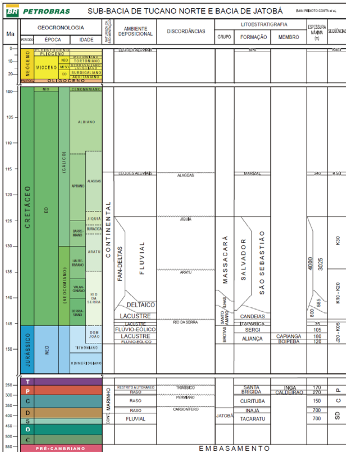
Figura 13 – Coluna estratigráfica da Sub-bacia de Tucano Norte e Jatobá (Costa et al., 2007).
