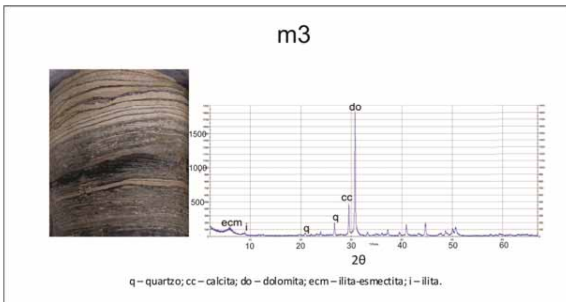
Figura 91 - Difratoograma mostrando delgados níveis de dolomito intercalados com níveis de folhelhos ricos em matéria orgânica, no topo do calcário peletoidal da microfácies m3 da UC1 (85,30-85,37m), do poço estratigráfico 2-JSN-01-PE (Vortisch et al. , 2011).
