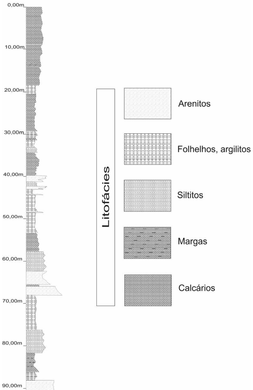
Figura 22 – Perfil Esquemático do Poço Estratigráfico 2–JSN–0-PE
