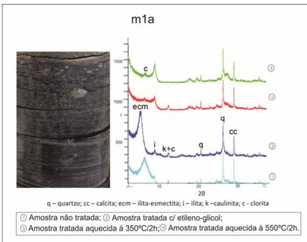
Figura 89 - Difratoograma do ritmo argilo-carbonático, microfácies m1a, da UC1 (84,77-84,84m), do poço estratigráfico 2-JSN-01-PE (Vortisch et al. , 2011).
