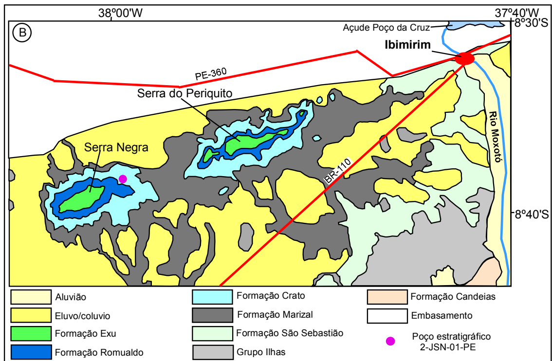
Figura 21 – Mapa Geológico Esquemático de parte da Bacia do Jatobá.
