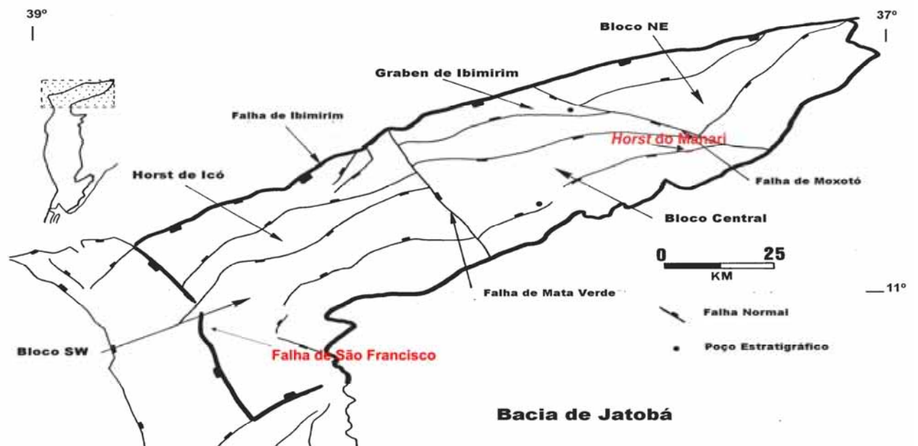
Figura 20 – Arcabouço estrutural da Bacia do Jatobá. Modificado de Magnavita, 1992 ( apud , Rocha & Leite, 1999).
