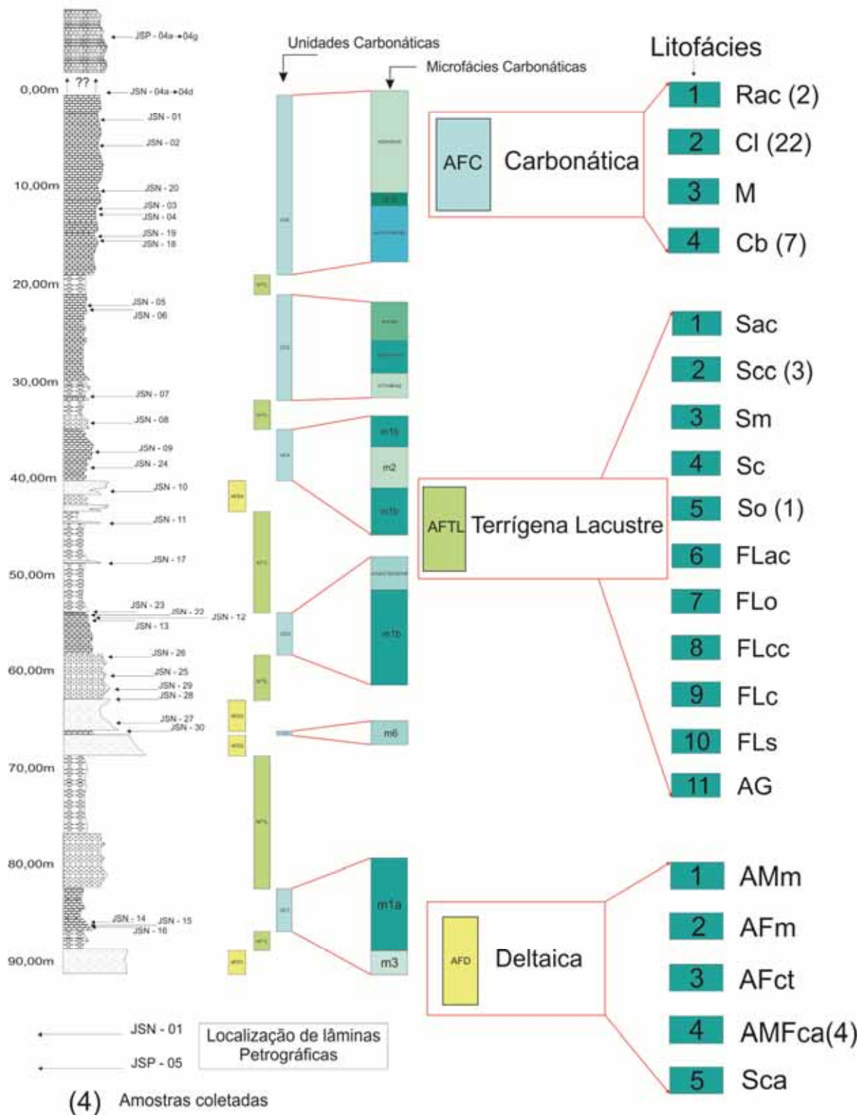
Figura 69 – Análises Petrográficas
