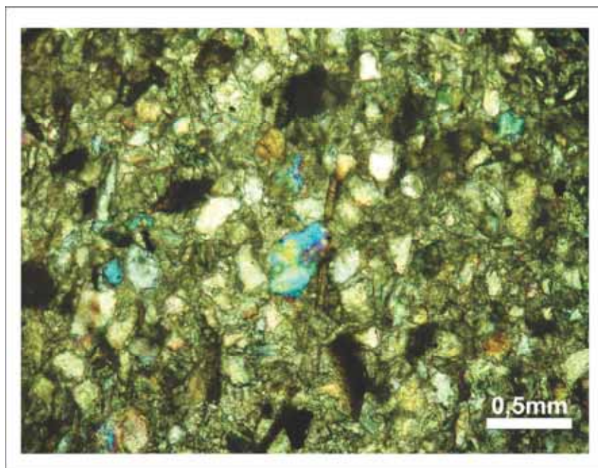
Figura 31 – Fotomicrografia (JSN-28) mostrando grãos angulosos de quartzo, em arenitos da litofácies AFm (NX).
