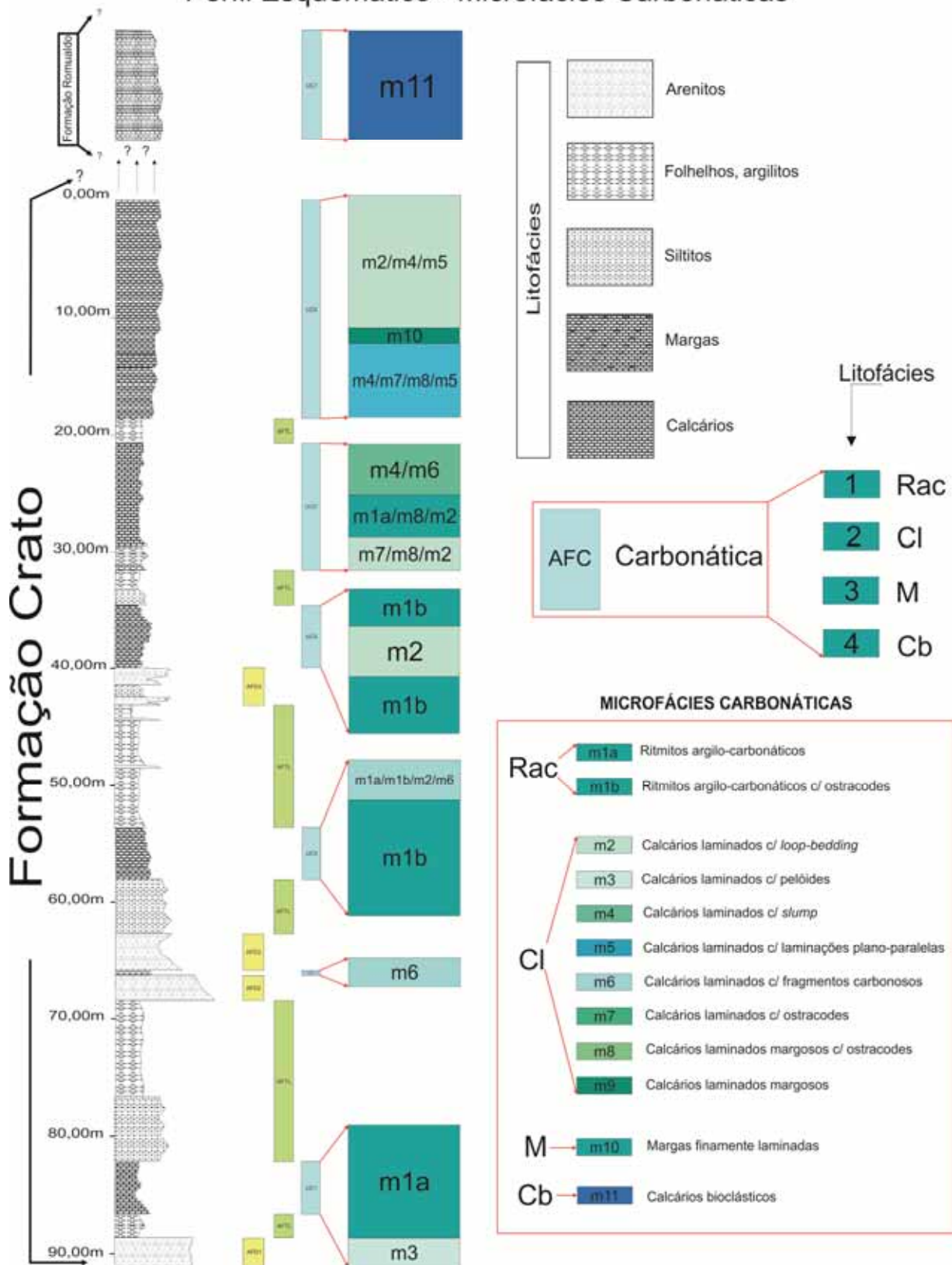
Figura 44 – Microfácies Carbonáticas
