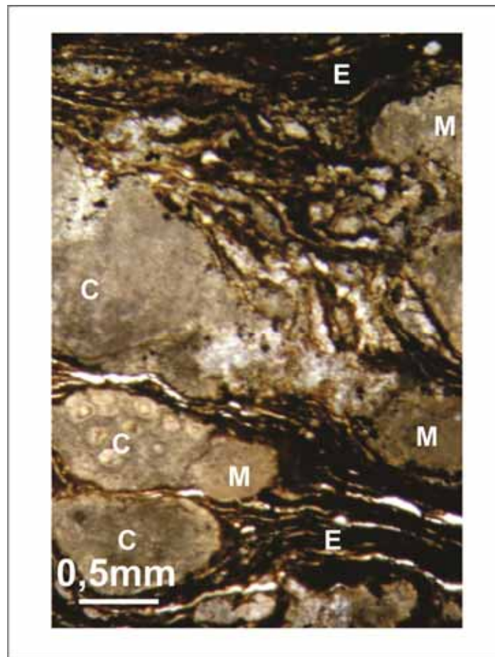
Figura 72 – Fotomicrografia (JSN-15) mostrando pelóides constituídos por calcisferas (C) e micrita (M), permeados por esteiras algálicas (E) em calcários da microfácies m3 (NX).
