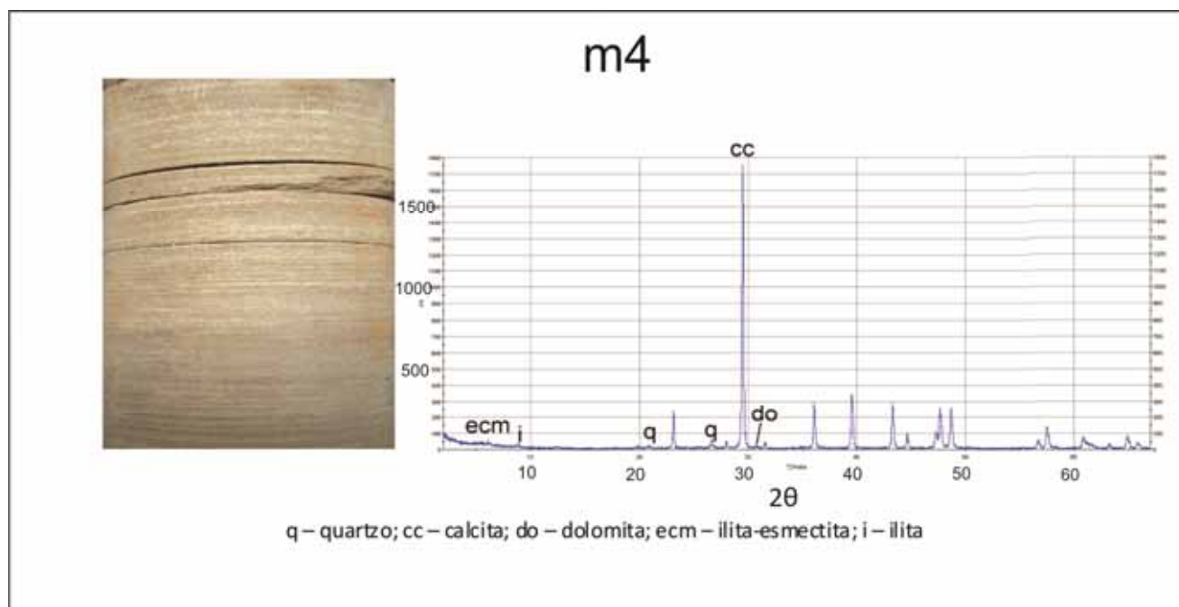
Figura 92 - Difratoograma do calcário laminado da microfácies m4 da UC5 (21,38-21,46m), parcialmente oxidado, com traços de dolomita e silicatos, do poço estratigráfico 2-JSN-01-PE (Vortisch et al. , 2011).
