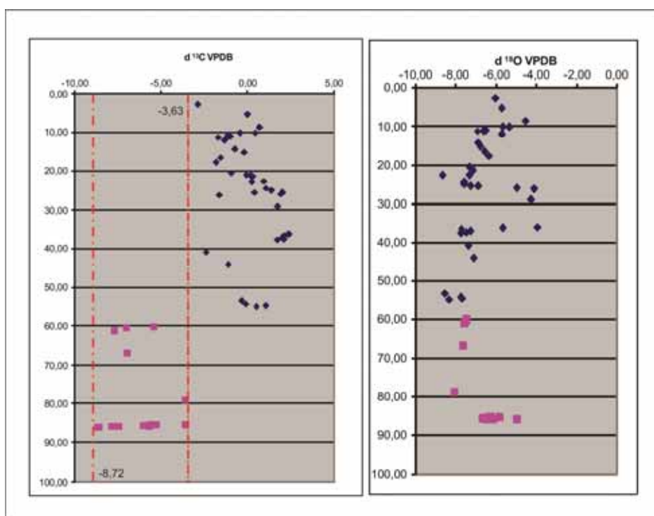
Figura 82 – Distribuição isotópica do Carbono e do Oxigênio, no poço 2-JSN-01-PE. Os valores em rosa são da porção inferior e os azuis da porção superior do poço.
