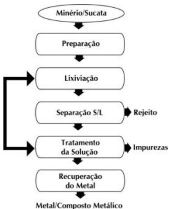
Figura 1 - Etapas principais de um fluxograma hidrometalúrgico
