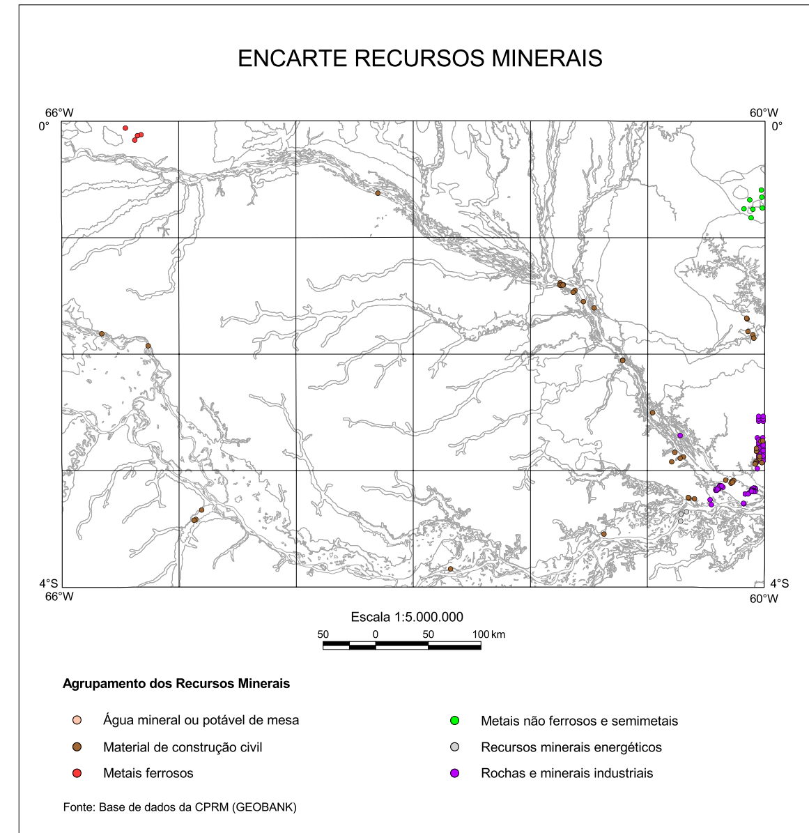
RELAÇÃO DE RECURSOS MINERAIS SELECIONADOS E REPRESENTADOS NA FOLHA MANAUS SA.20
