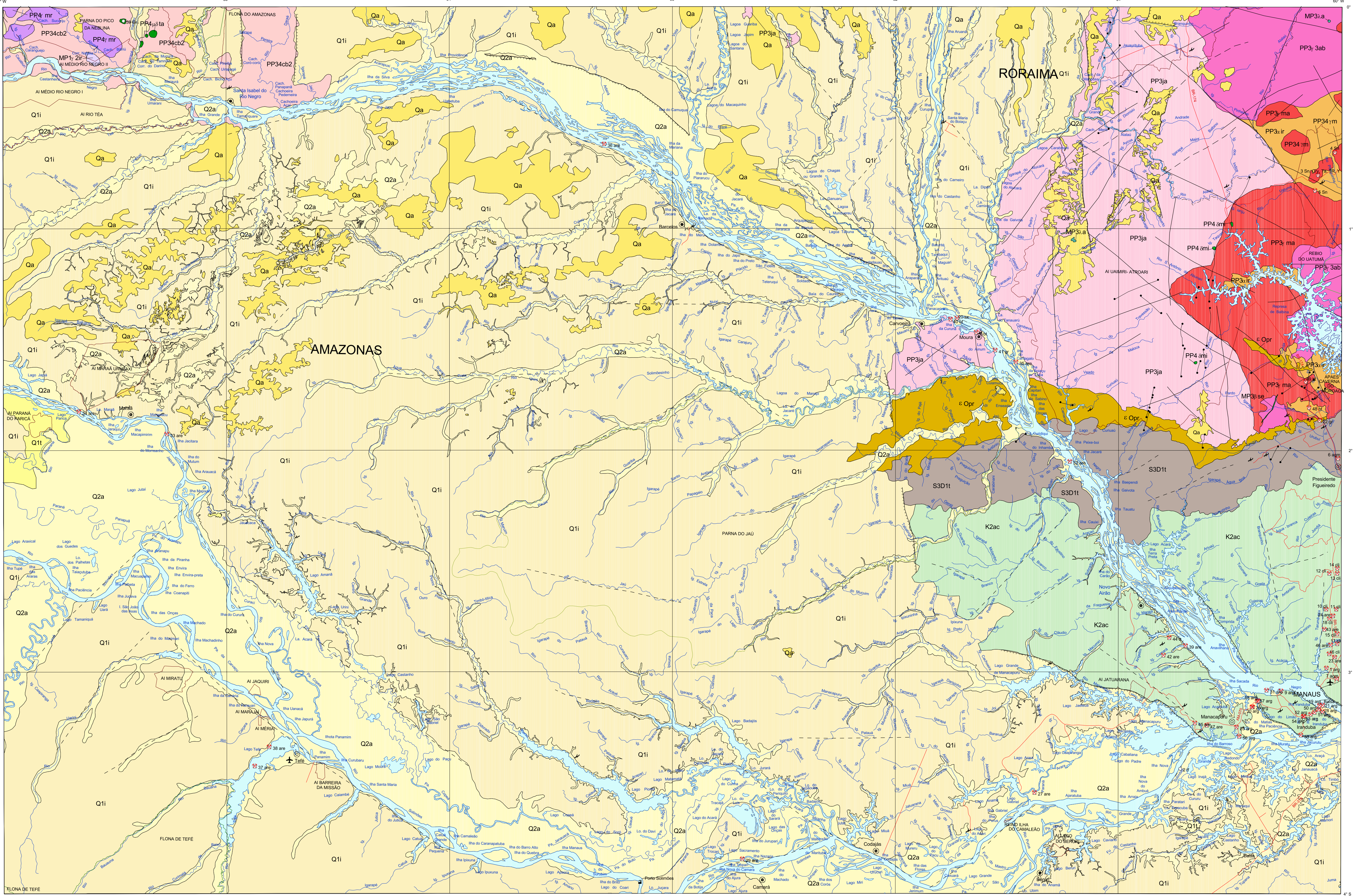
NOTAS: Todas as idades em milhões de anos. U/P = Ubatuba-Chumbé; P/Lu/P = Ourimbá-Chumbé. Valores de datações sedimentares em cor amarela indicam datas de cristalização.
