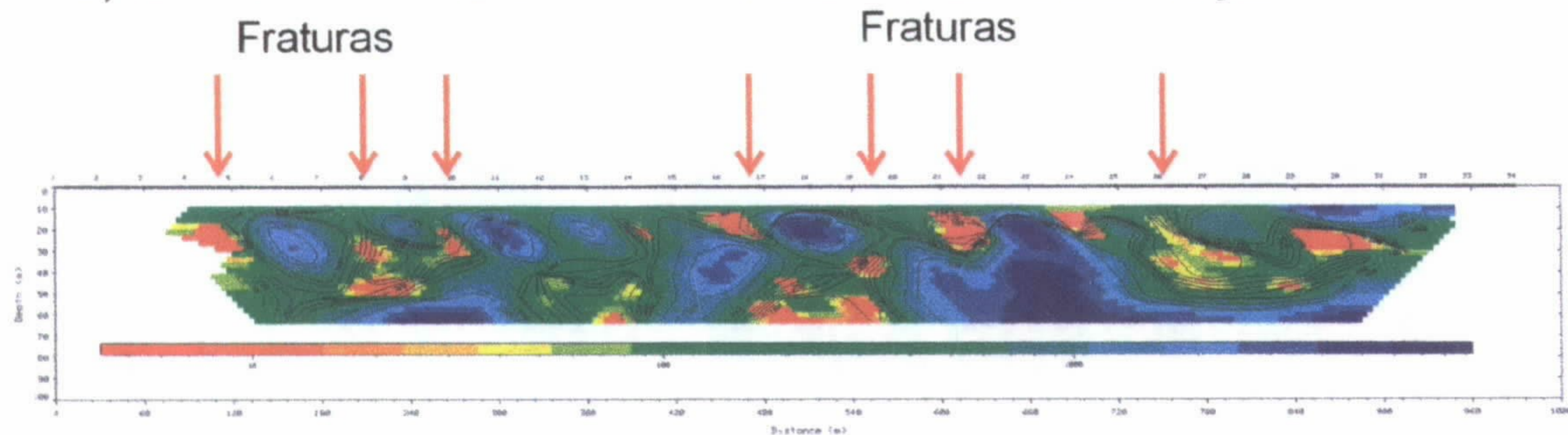
Figura 5 – Perfil com levantamento eletromagnético e de resistividade elétrica de Ponta da Várzea.
