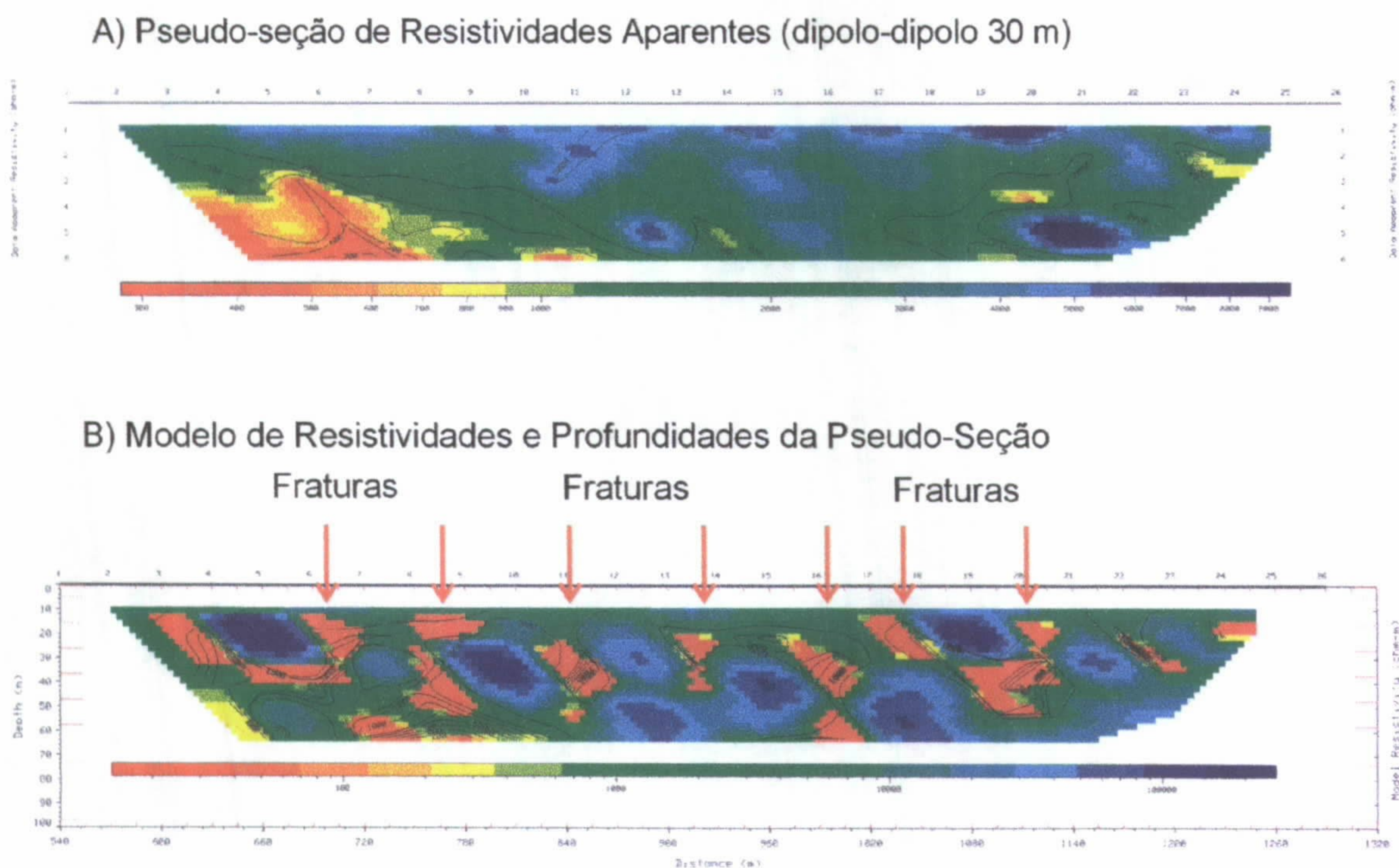
Figura 3 – Parte mediana do caminhamento de resistividade elétrica do perfil de Travessão.
