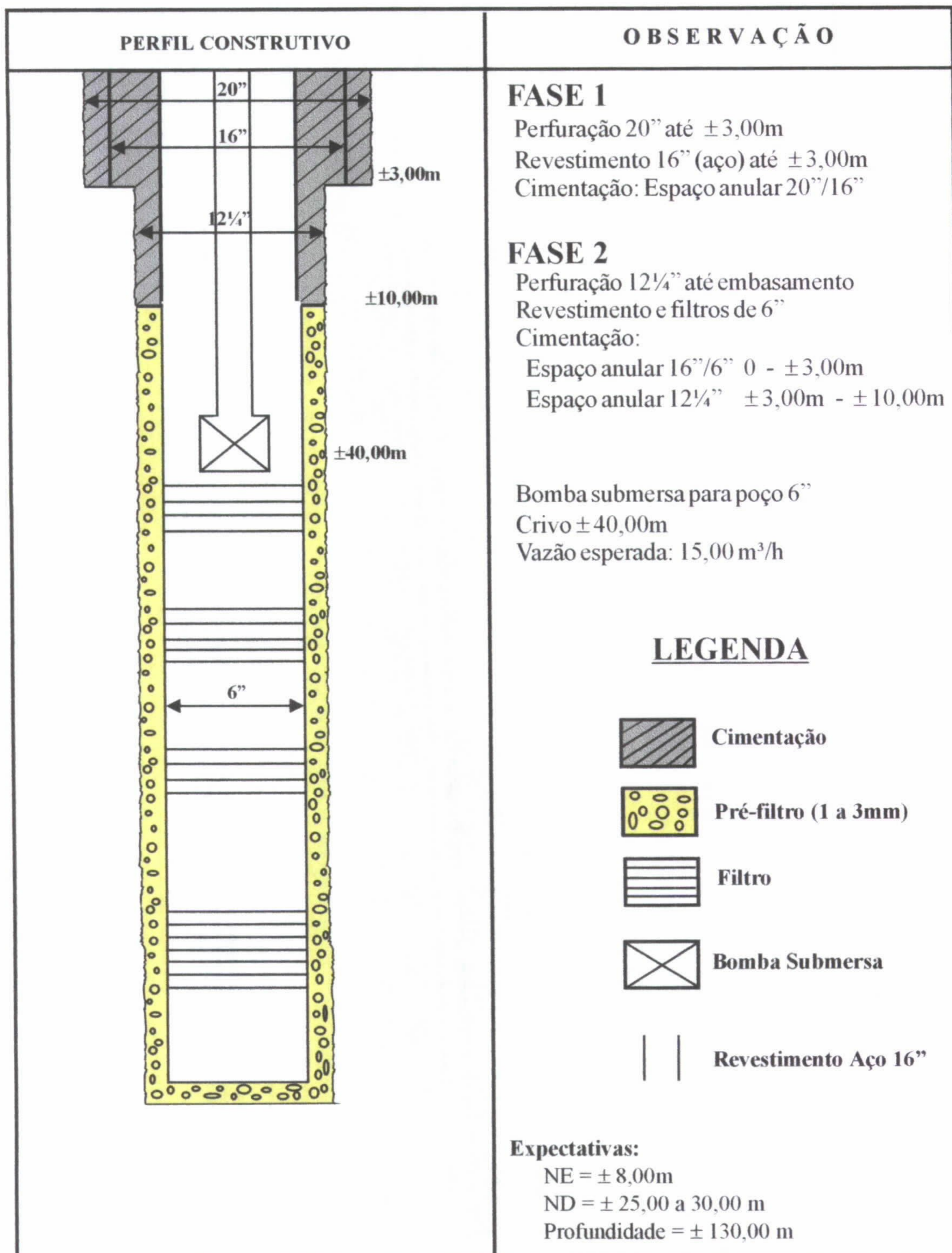
Figura 15 – Sugestão de perfil construtivo do poço tubular.
