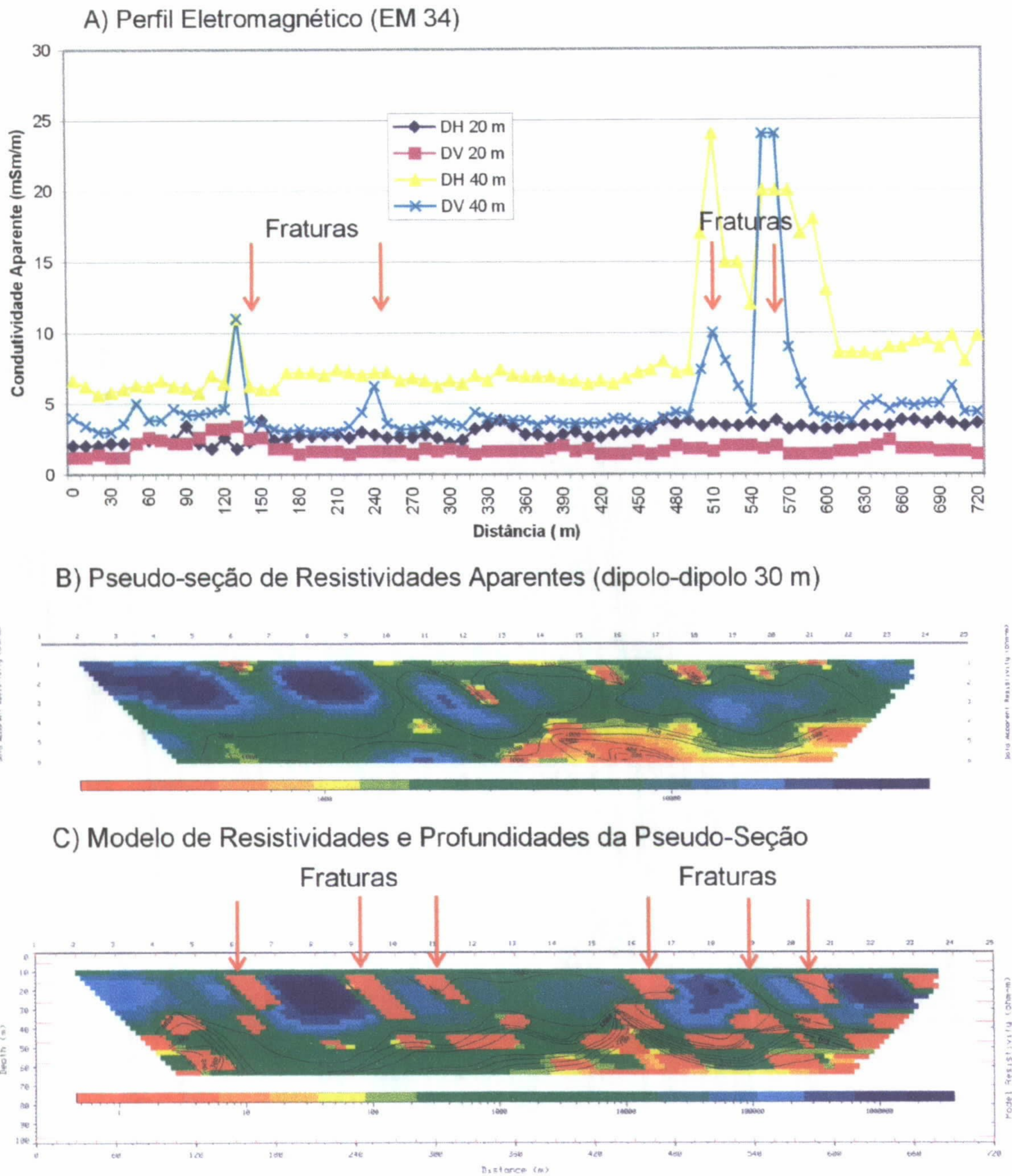
Figura 4 – Parte leste do levantamento eletromagnético e de resistividade elétrica do perfil de Catimbau.
