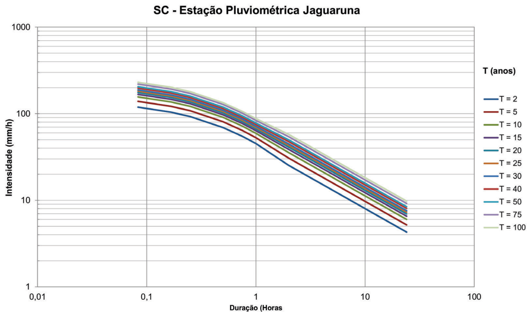
Figura 02 - Curvas intensidade-duração-frequência.
