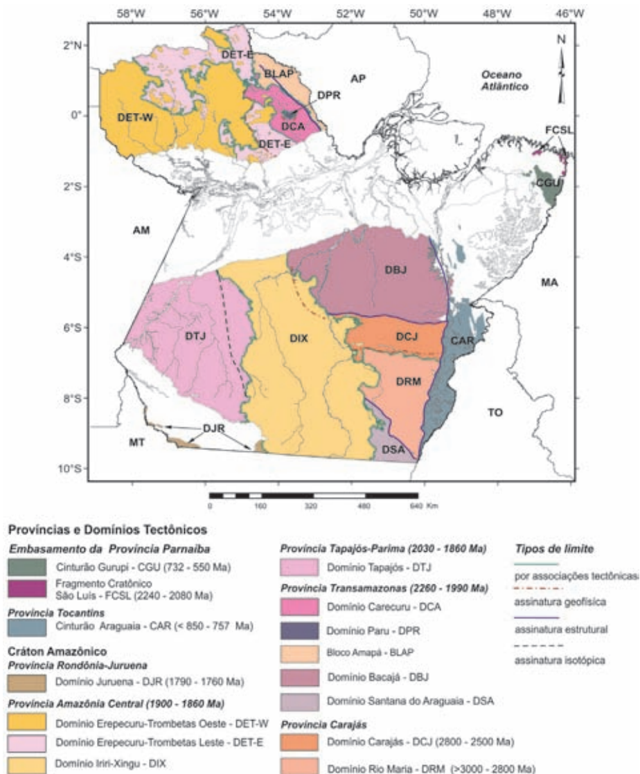
Figura 2.1 – Províncias e domínios tectônicos do estado do Pará. Fonte: Vasquez e Rosa-Costa (2008).
