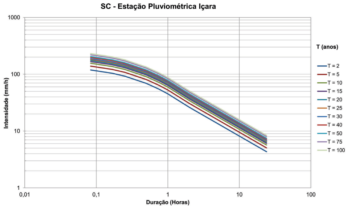
Figura 02 - Curvas intensidade-duração-frequência.
