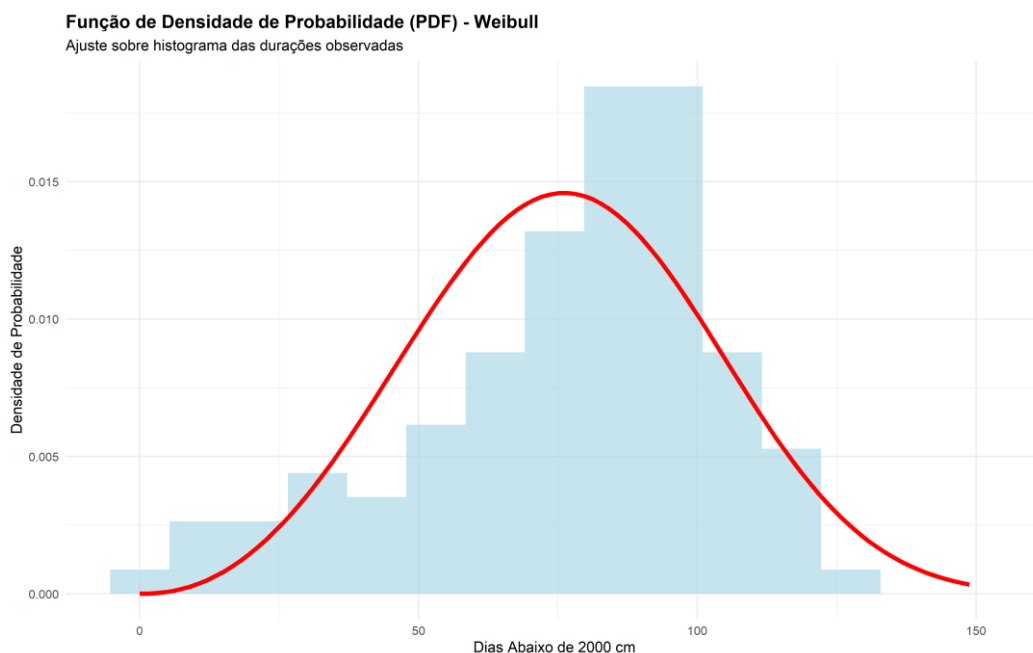
Figura 4.1: Ajuste da distribuição Weibull à duração de eventos de estiagem (dias abaixo de 20 m).
