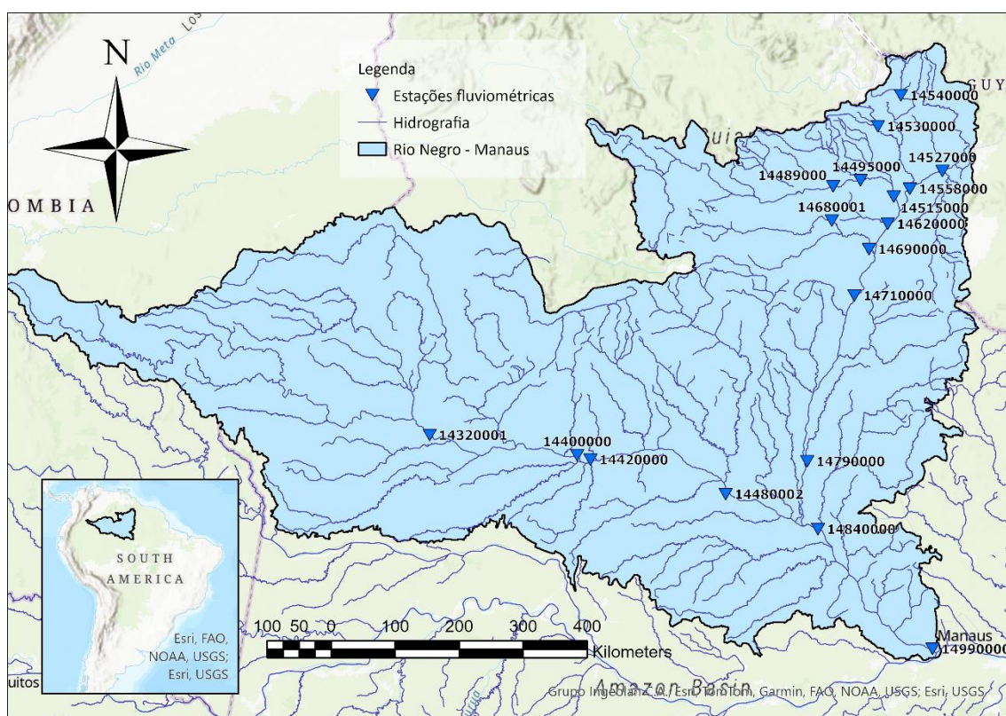
Figura 1.1: Bacia do rio Negro até a estação Manaus (14990000).
