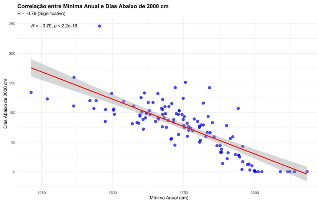
Figura 4.3: Análise de correlação entre os níveis mínimos anuais e o número de dias que o rio fica abaixo da cota de 20 m. A correlação significativa ( p -valor < 0,05 ) indica que quanto mais baixo o nível que o rio atinge em um determinado ano, mais tempo ele permanece em níveis baixos.
