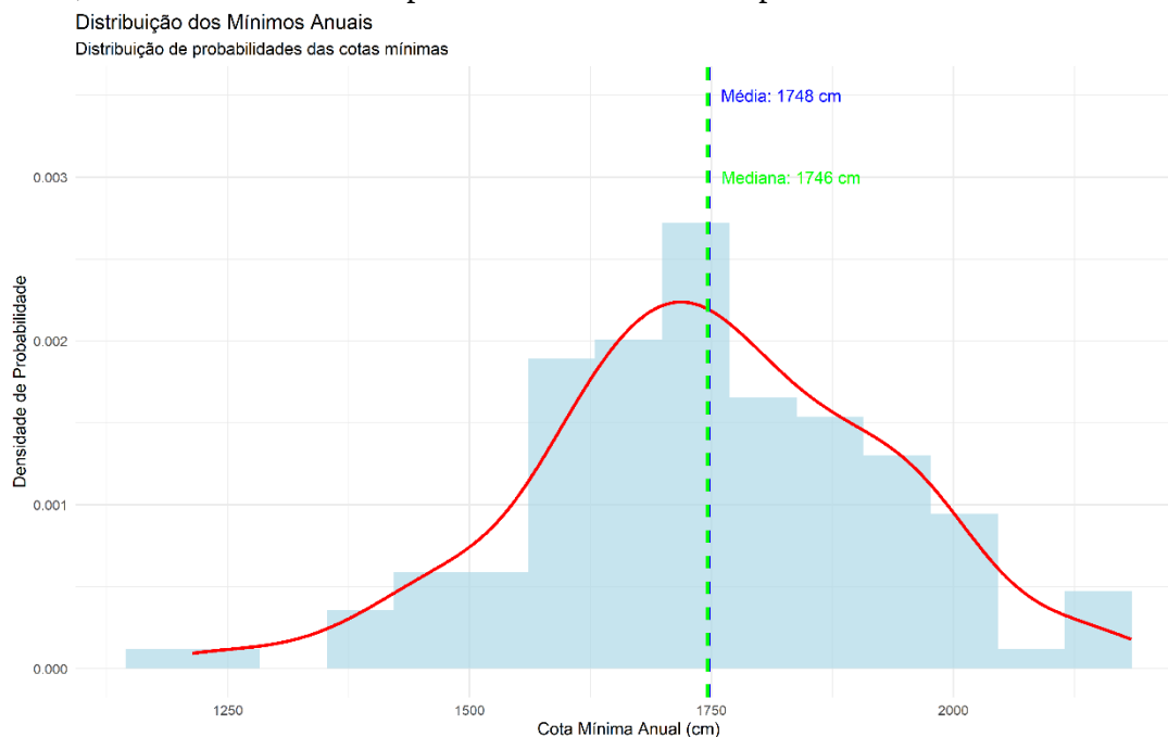
Figura 3.3: Ajuste da distribuição normal aos dados de mínimas anuais na estação Manaus
