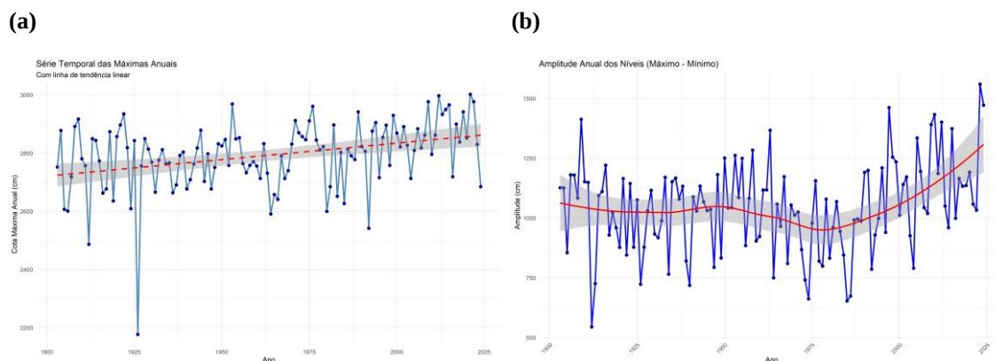
Figura 3.2: Tendência temporal das (a) máximas anuais e da (b) amplitude de variação anual na estação de Manaus. A linha de regressão linear (vermelha) indica uma significativa taxa de aumento tanto da máxima quanto da amplitude. No caso da tendência de aumento das máximas, ela aumentou a uma taxa de 1,1 cm/ano ao longo do período 1903-2025. A tendência da amplitude também é cíclica, a exemplo das mínimas, contudo depois de 1970 a taxa média de aumento foi de 7,6 cm/ano.
