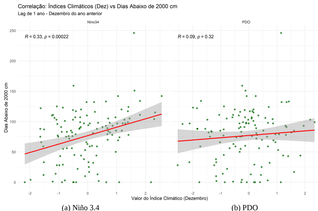
Figura 5.5: Correlação entre os índices climáticos de dezembro do ano anterior e a duração dos eventos de baixa vazão na estação de Manaus. Índice Niño 3.4 (a): correlação positiva significativa ( R = 0,33 ; p = 0,0002 ); Índice PDO (b): sem correlação significativa ( R = 0,09 ; p = 0,32 ).
