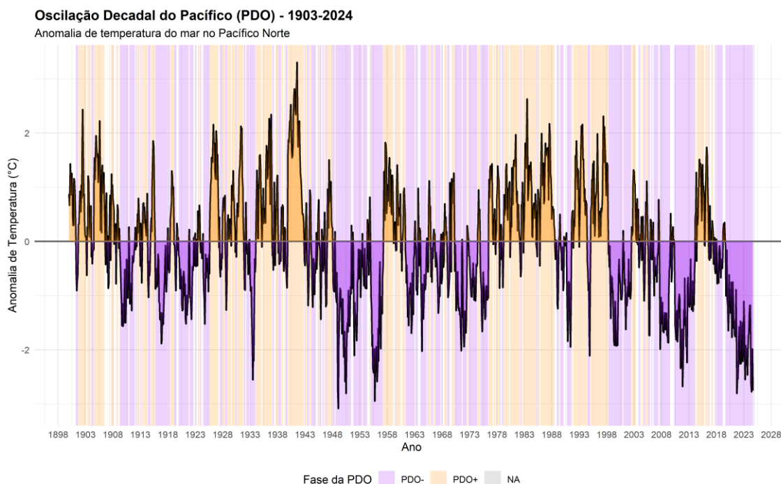
Figura 5.3: Série temporal da Oscilação Decadal do Pacífico (PDO) no período 1903-2024. O gráfico mostra a anomalia de temperatura da superfície do mar no Pacífico Norte, representando as fases positiva (PDO+) e negativa (PDO-) da oscilação. As bandas laranja indicam fases quentes (PDO+), enquanto as bandas roxas representam fases frias (PDO-). Ressalte-se que o período atual apresenta uma situação de PDO negativo.
