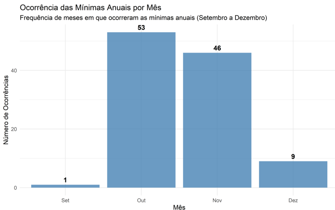
Figura 2.3: Distribuição mensal de ocorrência das mínimas anuais
