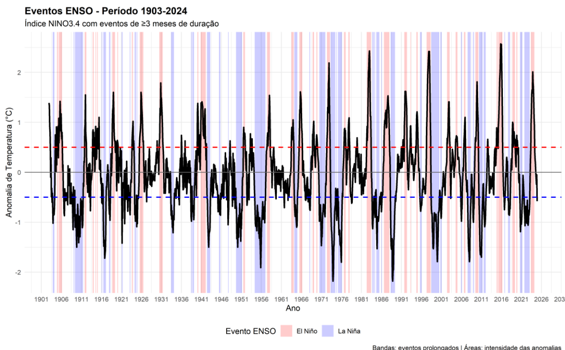
Figura 5.2: Evolução temporal do índice ENSO (El Niño-Oscilação Sul) no período 1903-2024. O gráfico apresenta a anomalia de temperatura da superfície do mar na região NINO3.4 do Pacífico Central. As bandas coloridas destacam os eventos de El Niño (vermelho) e La Niña (azul) que persistiram por pelo menos 3 meses consecutivos acima dos limiares de \pm 0,5^{\circ}\text{C} . A linha preta contínua mostra a variação mensal do índice. Ressalte-se que o período atual apresenta uma situação de neutralidade.
