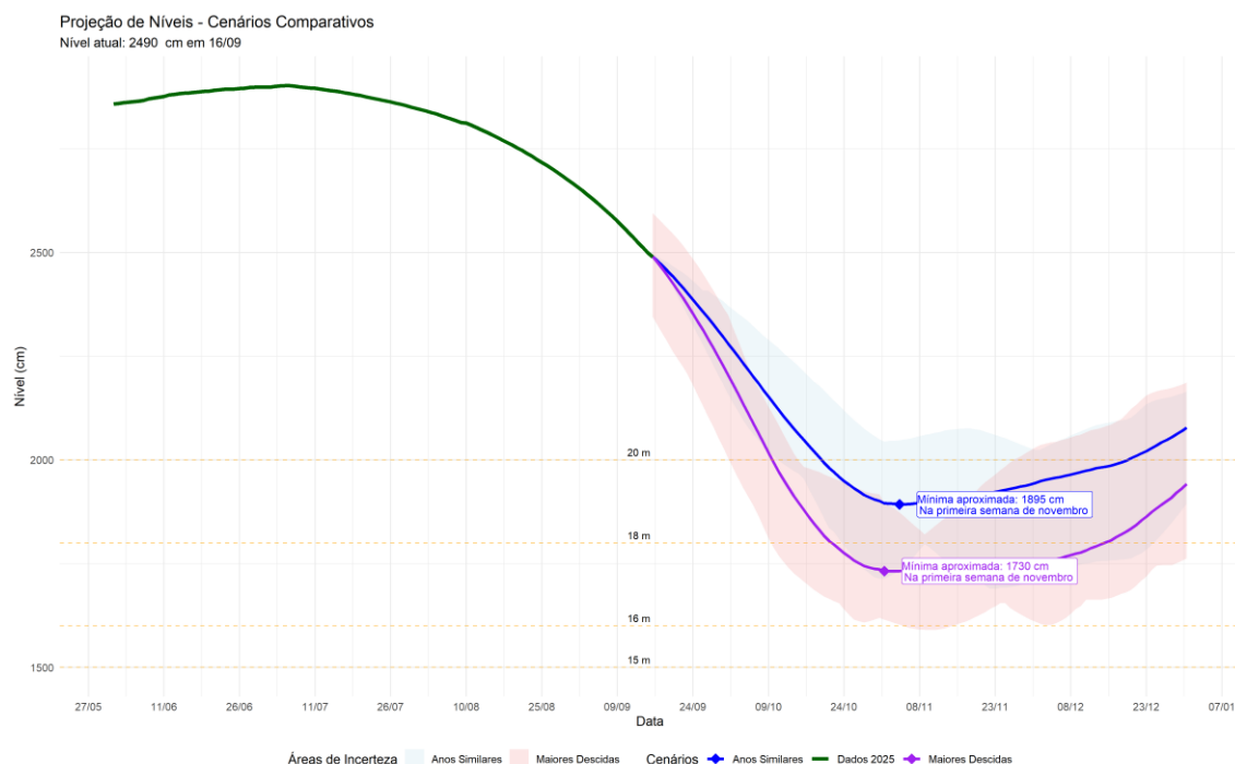
Figura 5.1: Projeção comparativa do nível d'água em Manaus a partir de 16/09/2025 - Simulação do comportamento futuro do nível (em cm) com base no patamar atual de 2490 cm. Apresenta a projeção derivada de anos históricos similares (Anos Similares) e o cenário de maiores descidas registradas (Maiores Descidas). As faixas sombreadas representam os envelopes de incerteza das projeções.
