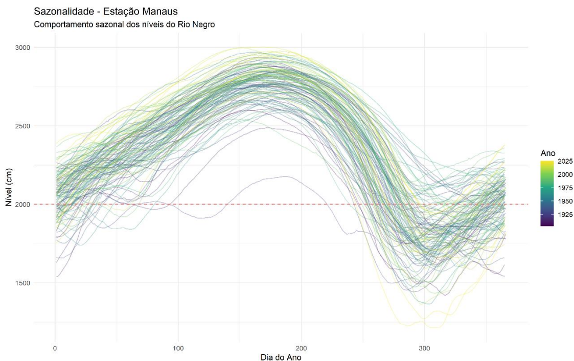
Figura 2.2: Sazonalidade dos níveis do rio Negro na estação Manaus.
