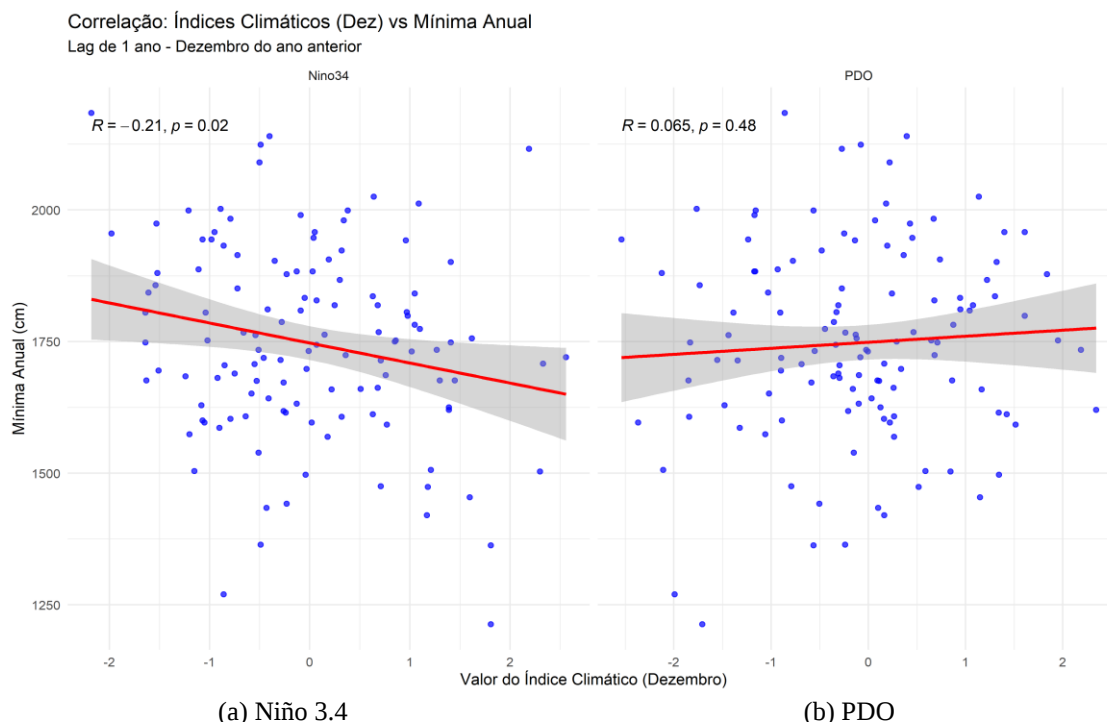
Figura 5.4: Correlação linear entre os índices climáticos do mês de dezembro do ano anterior e o nível mínimo anual observado na estação de Manaus. O índice Niño 3.4 (a) mostra uma correlação negativa moderadamente significativa ( R = -0,21 ; p = 0,02 ) com a vazante do ano seguinte, enquanto a PDO (b) não apresentou uma correlação significativa ( R = 0,065 ; p = 0,48 ) para o mesmo período.
