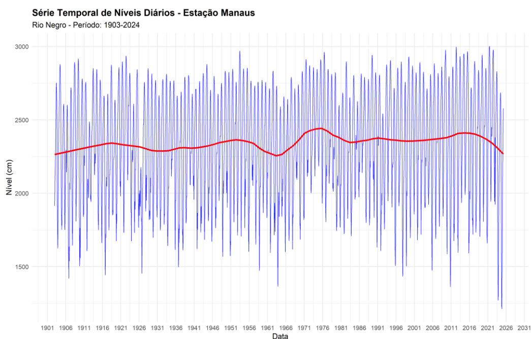
Figura 2.1: Série histórica de níveis médios diários na estação de Manaus entre 1903 e 2024. A linha vermelha indica a tendência de longo prazo ajustada por meio de regressão polinomial local (loess).
