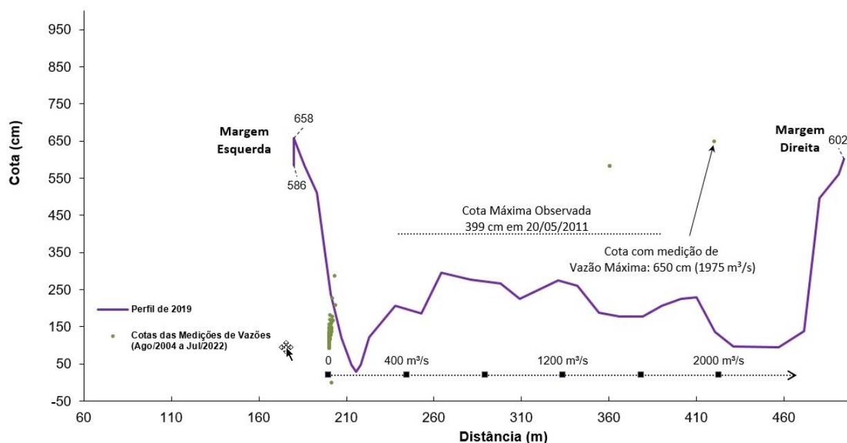
Figura 03 – Perfil da seção transversal da seção de réguas de Diba - Sítio Canto Alegre. Falha de leitura em 2008 e 2009 implicou na ausência de registro de cotas máximas observadas acima da cota associada à vazão máxima medida. Fonte: elaborado pelos autores.
