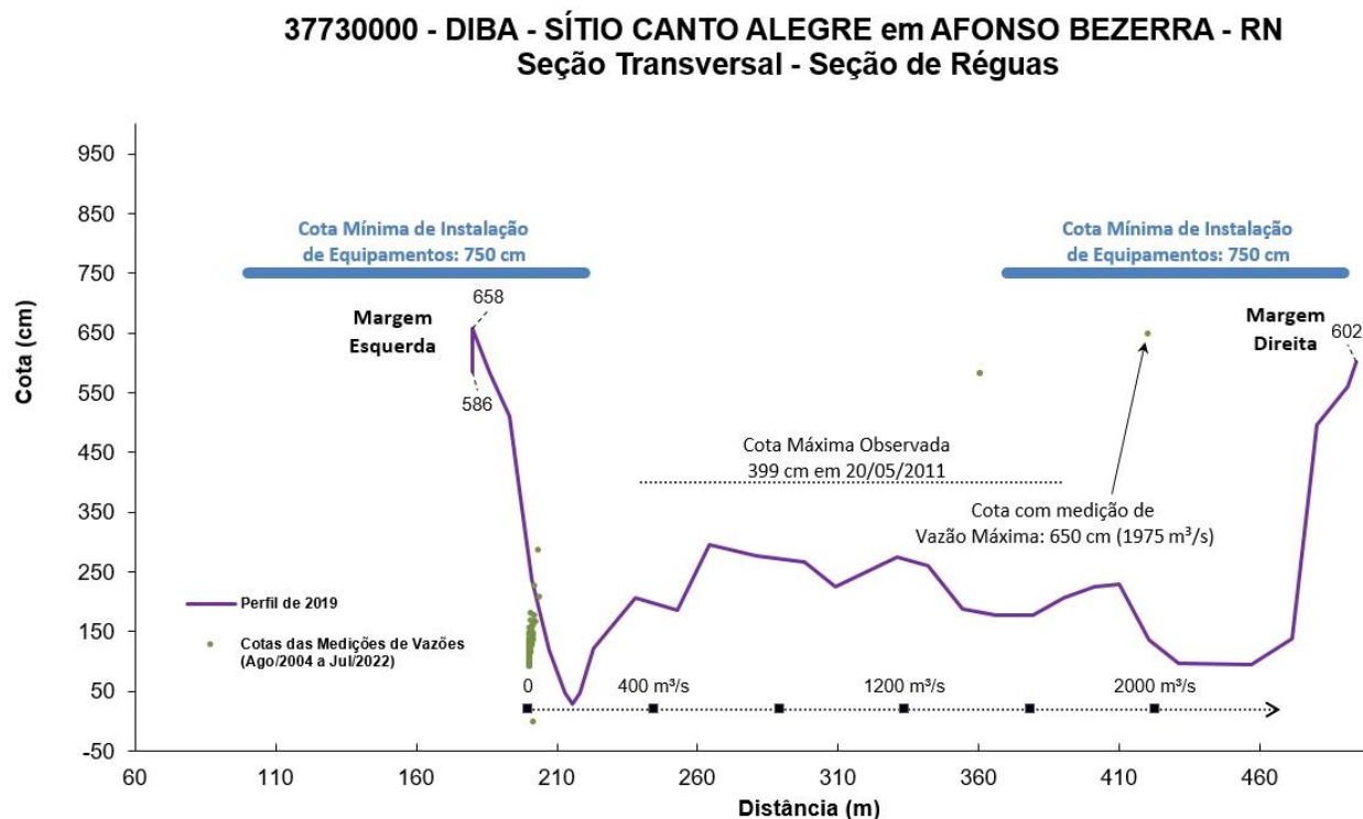
Figura 05 – Cota mínima de instalação de equipamentos. Falha de leitura em 2008 e 2009 implicou na ausência de registro de cotas máximas observadas acima da cota associada à vazão máxima medida. Fonte: elaborado pelos autores.
