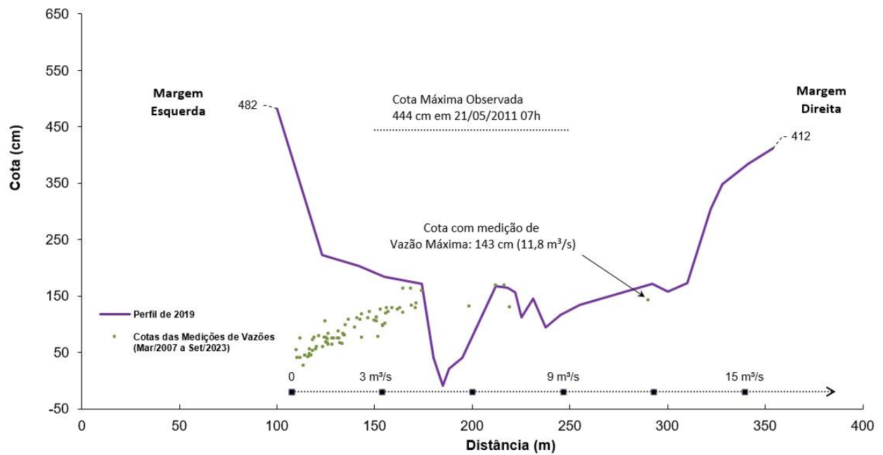
Figura 03 – Perfil da seção transversal da seção de régua de Alto Rodrigues. Fonte: elaborado pelos autores.
