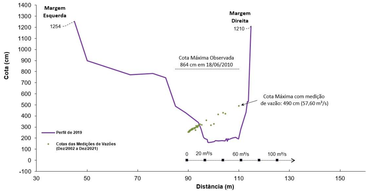
Figura 03 – Perfil da seção transversal da seção de régua de José Mariano. Fonte: elaborado pelos autores.
