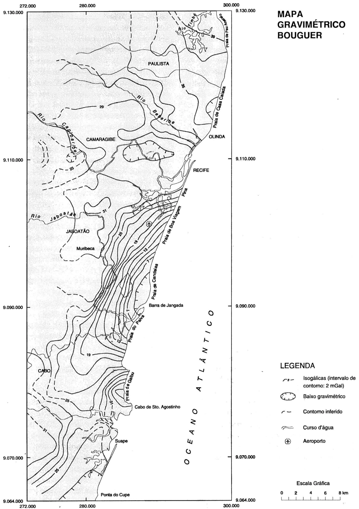
Figura 3 - Mapa gravimétrico Bouguer
