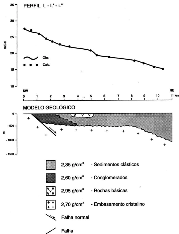
Figura 11 - Modelagem do perfil L-L'-L''
