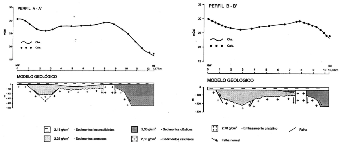
Figura 7 - Modelagem dos perfis A-A' e B-B'
