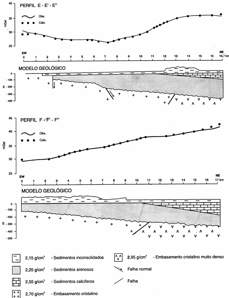
Figura 9 - Modelagem dos perfis E-E'-E'' e F-F'-F''
