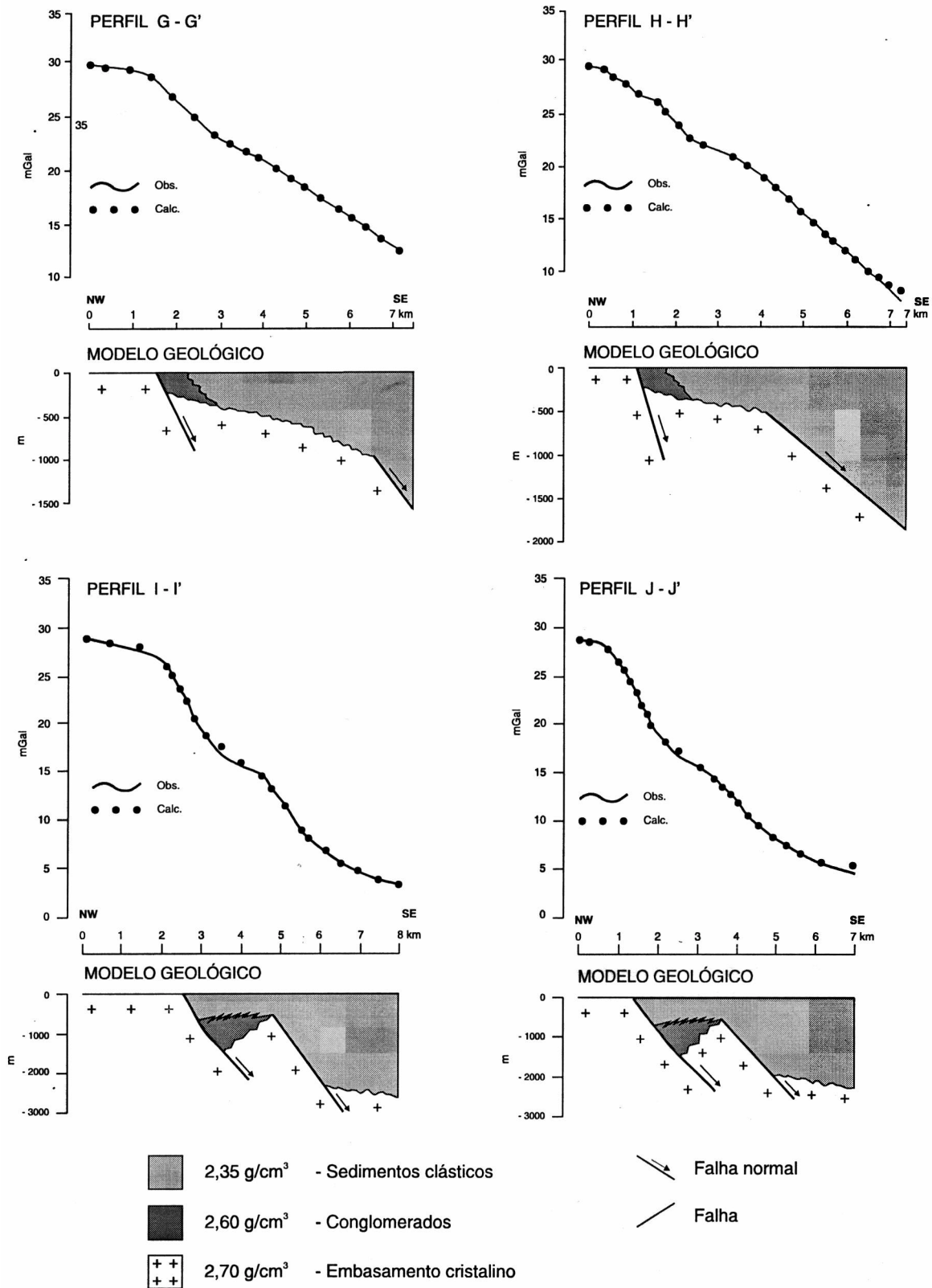
Figurta 10 - Modelagem gravimétrica dos perfis G-G', H-H', I-I' e J-J'
