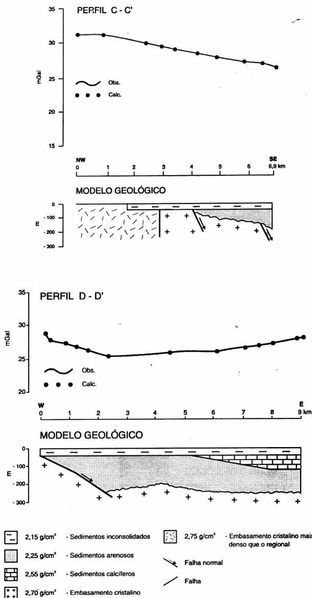
Figura 8 - Modelagem dos perfis C-C' e D-D'
