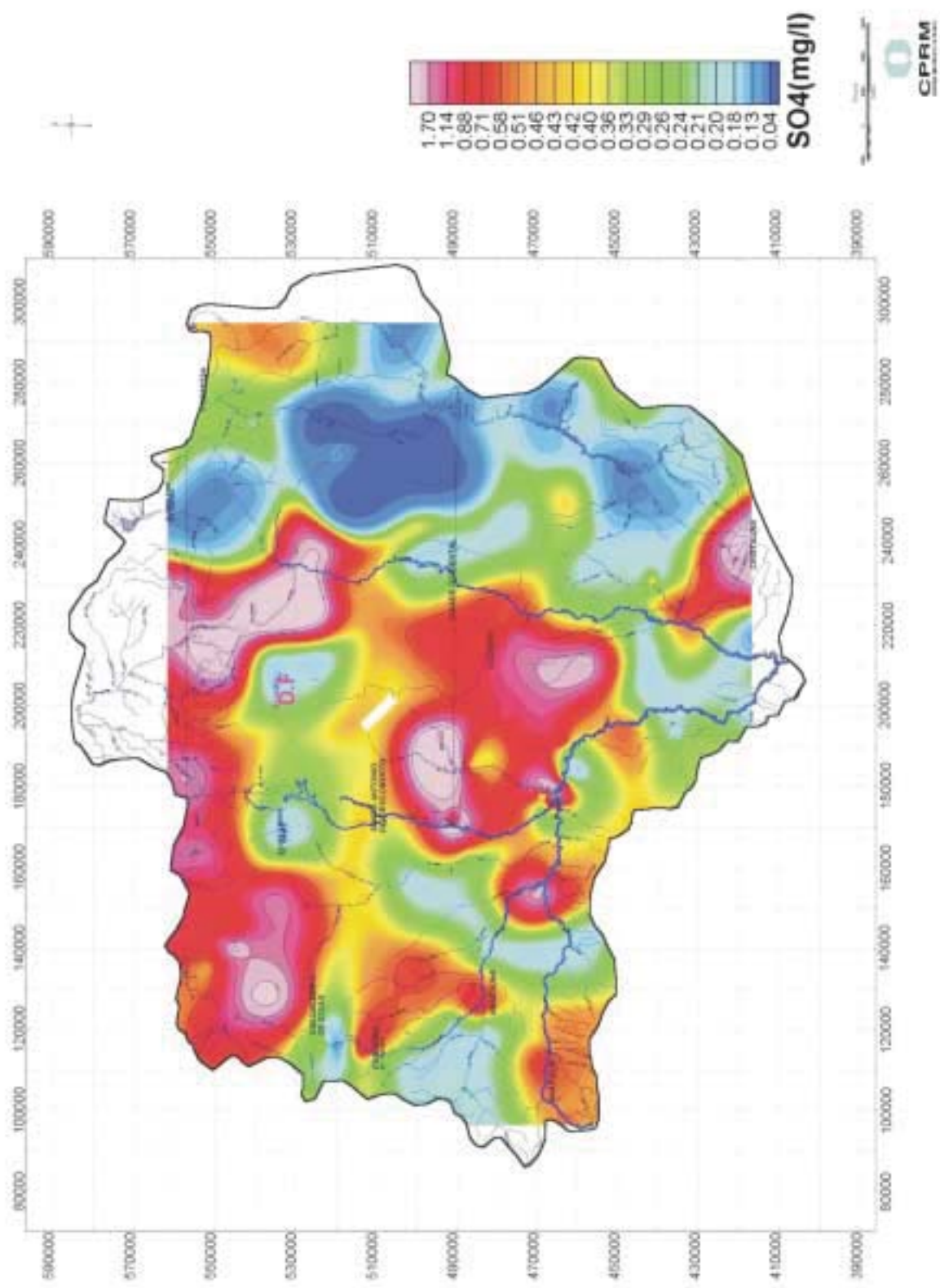
Figura 9.21 – Mapa interpretativo do sulfato em amostras de água (fase regional).
