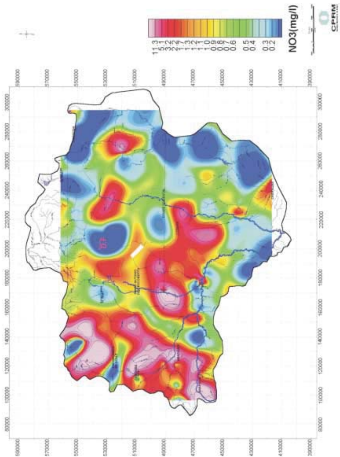
Figura 9.19 – Mapa interpretativo do nitrato em amostras de água (fase regional).
