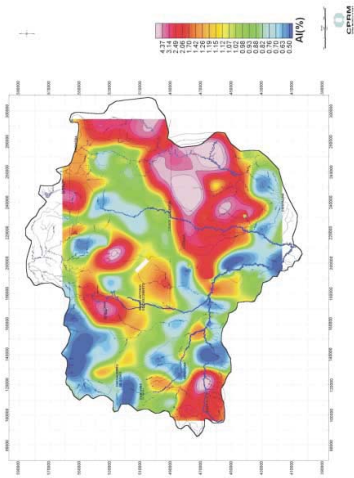
Figura 9.13 – Mapa interpretativo do alumínio em sedimentos de corrente.
