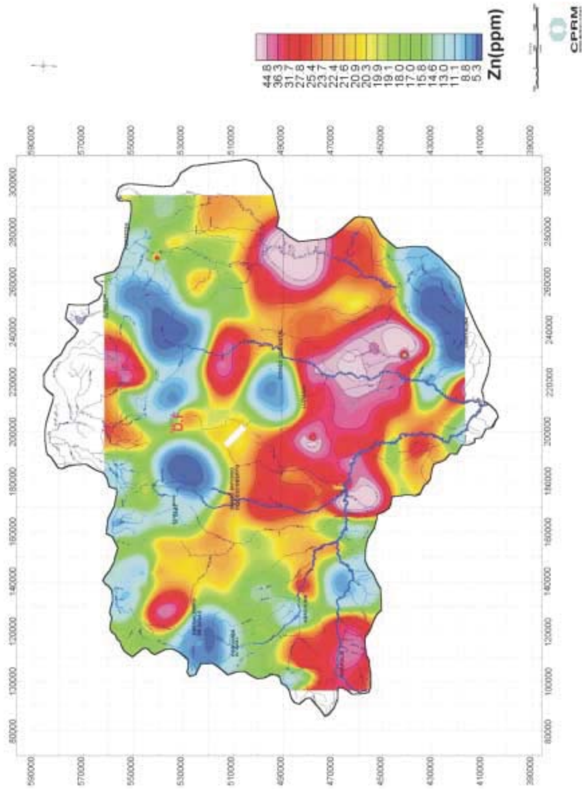
Figura 9.18 – Mapa interpretativo do zinco em sedimentos de corrente.
