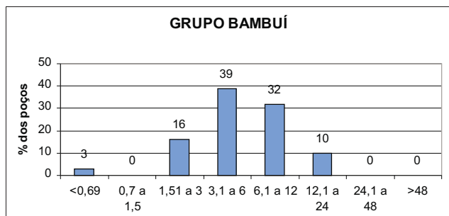
Figura 11.6 – Distribuição dos poços por faixa de vazão (m 3 /h).
