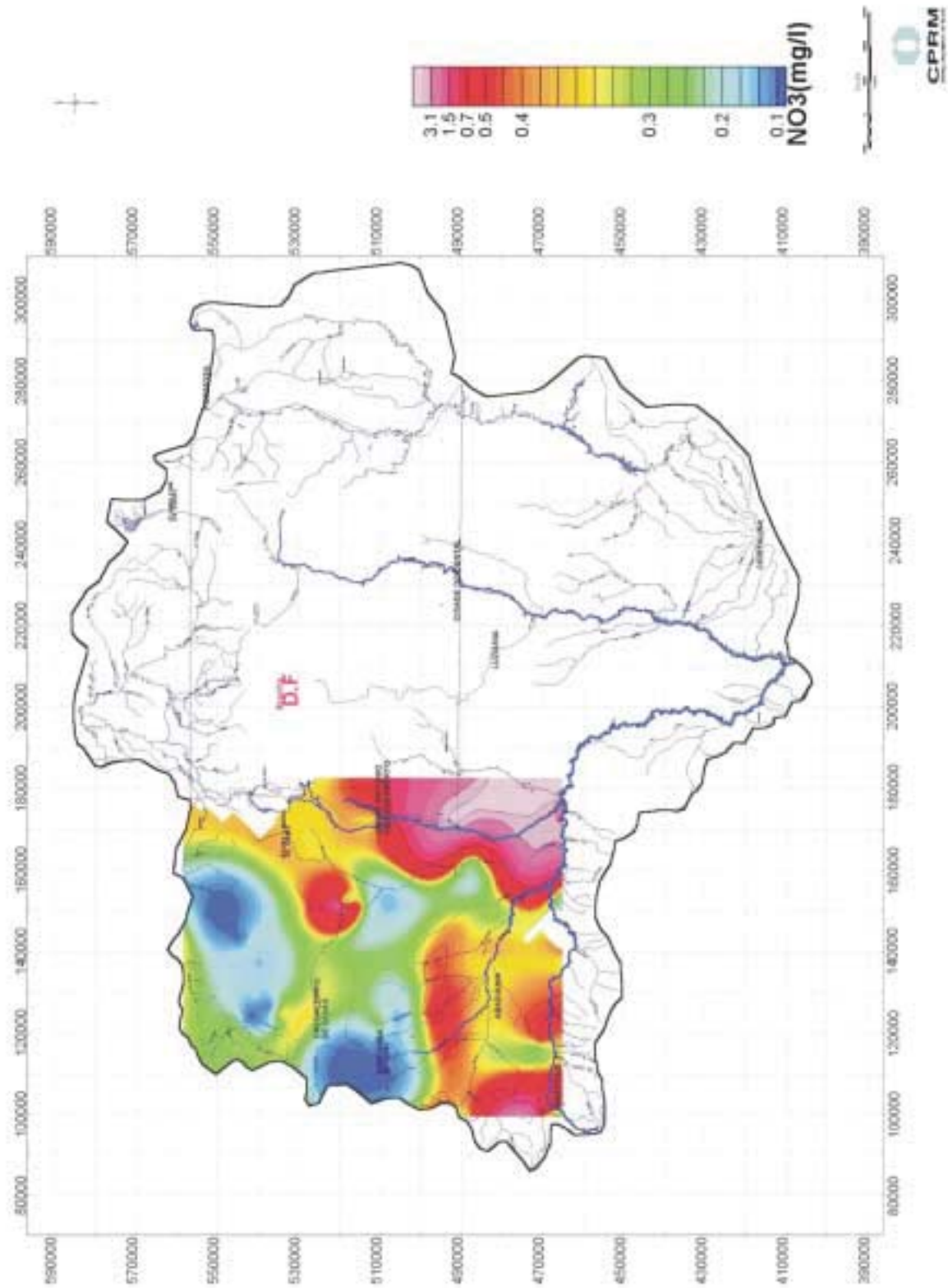
Figura 9.20 – Mapa interpretativo do nitrato em amostras de água (fase de verificação).
