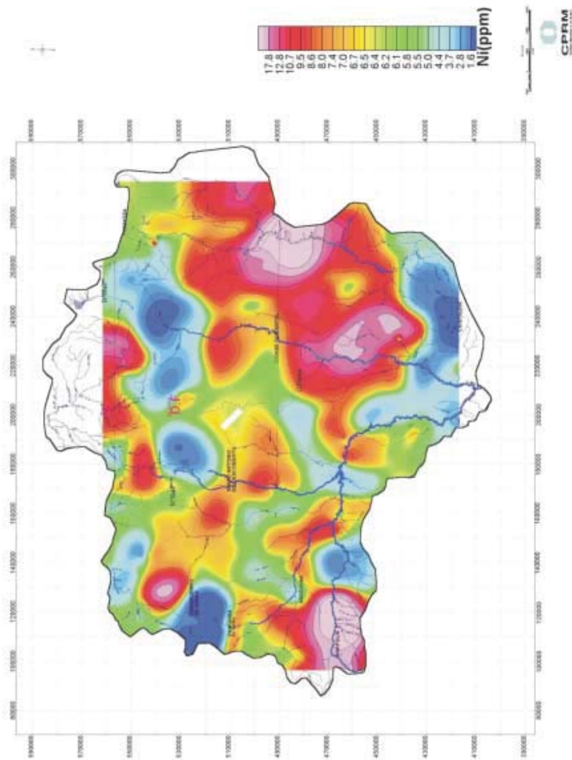
Figura 9.5 – Mapa interpretativo do níquel em sedimentos de corrente.
