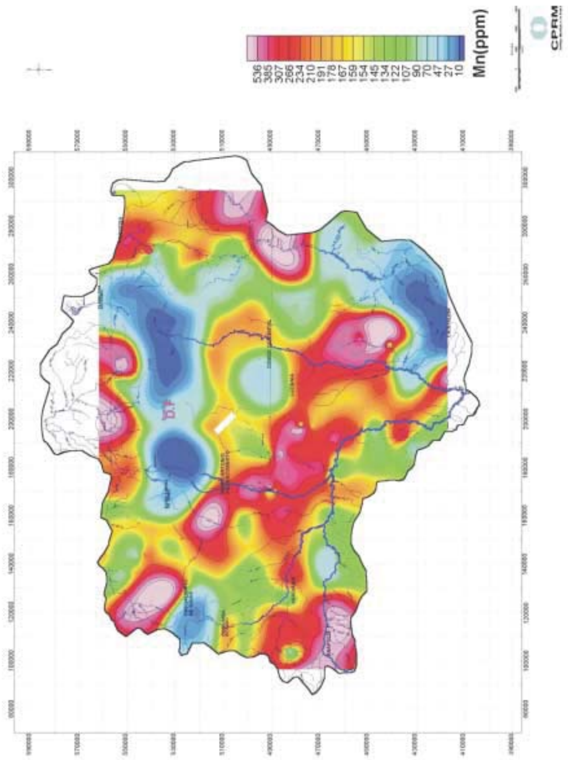
Figura 9.15 – Mapa interpretativo do manganês em sedimentos de corrente.
