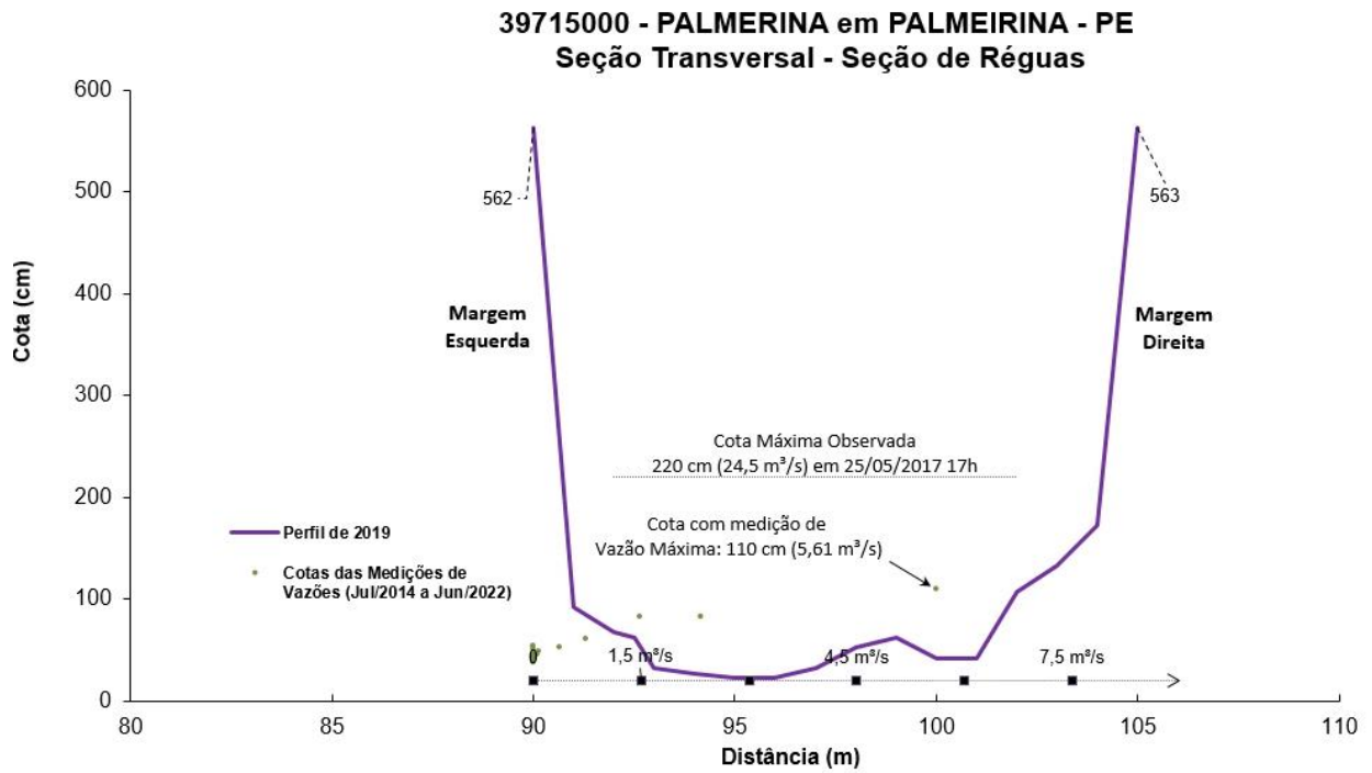
Figura 03 – Perfil da seção transversal da seção de régua de Palmeirina. Fonte: elaborado pelos autores.
